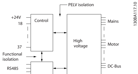
图 8.1 PELV 绝缘
