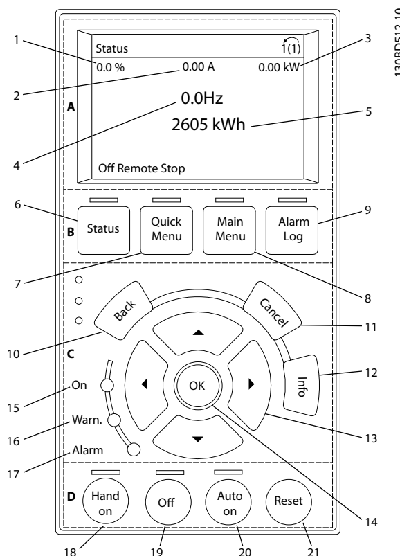
Ilustrația 5.1 Panou de comandă local (LCP)
