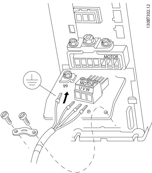
Ilustrația 4.6 Conexiunea motorului pentru tipul de carcasă A2 și A3
