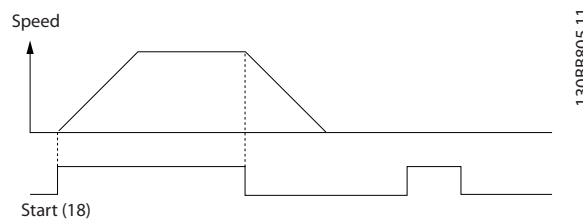
Ilustracja 6.2 Polecenie Start/stop z Bezpiecznym stopem
