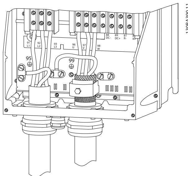
Ilustracja 4.8 Okablowanie silnika, zasilania i uziemienia dla typów obudów B i C wykonane kablem ekranowanym
