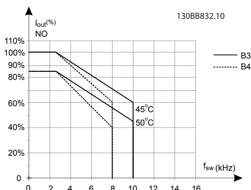
Illustration 9.11 Déclassement de I_{\text{sortie}} pour différentes T_{\text{AMB, MAX}} pour protections de types B3 et B4, utilisant SFAVM en mode surcharge normale (surcouple de 110 %)
