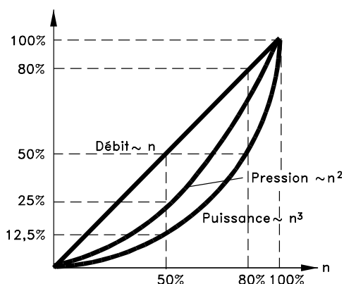
Illustration 2.10 Rapport entre débit, pression et puissance consommée en tr/min
