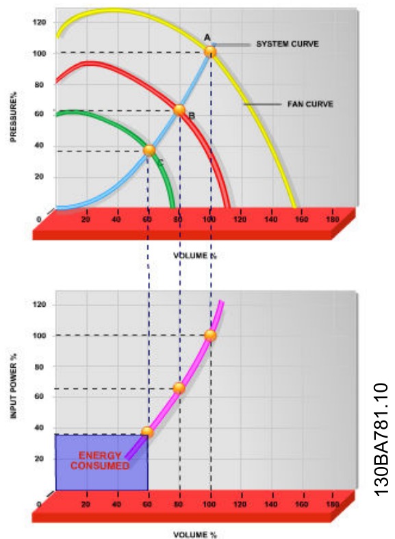
Illustration 2.9 Lors de l'utilisation d'un variateur de fréquence pour diminuer la capacité du ventilateur à 60 %, des économies d'énergie de plus de 50 % peuvent être obtenues dans des applications typiques.
