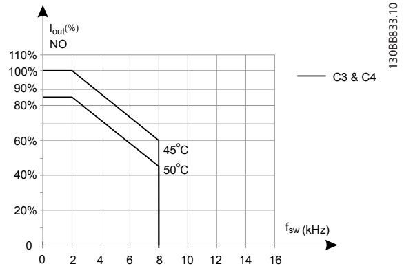
Illustration 9.19 Déclassement de I sortie pour différentes T AMB , MAX pour protections de types C3 et C4, utilisant SFAVM en mode surcharge normale (surcouple de 110 %)
