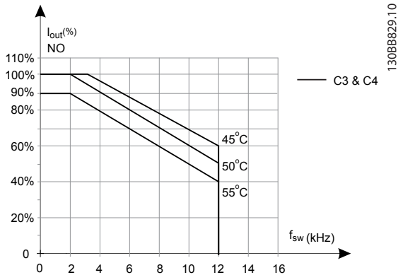
Illustration 9.17 Déclassement de I sortie pour différentes T AMB , MAX pour protections de types C3 et C4, utilisant 60° AVM en mode surcharge normale (surcouple de 110 %)
