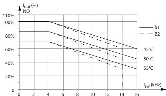
Illustration 9.8 Déclassement de I_{\text{sortie}} pour différentes T_{\text{AMB, MAX}} pour protections de types B1 et B2, utilisant 60^\circ AVM en mode couple normal (surcouple de 110 %)
