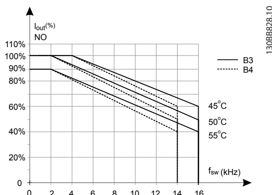
Illustration 9.9 Déclassement de I_{\text{sortie}} pour différentes T_{\text{AMB, MAX}} pour protections de types B3 et B4, utilisant 60^\circ AVM en mode surcharge normale (surcouple de 110 %)
