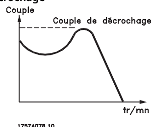
Illustration 1.1 Couple de décrochage
