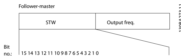
Illustration 8.17 Mot d'état
