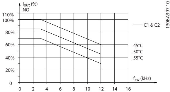
Illustration 9.16 Déclassement de I sortie pour différentes T AMB , MAX pour protections de types C1 et C2, utilisant 60° AVM en mode surcharge normale (surcouple de 110 %)
