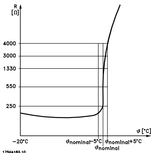
Illustration 2.41 Déclenchement de la thermistance
