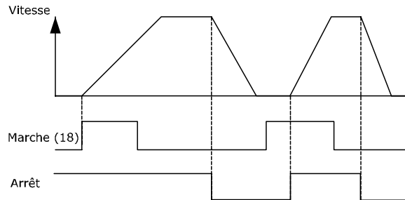
Illustration 6.54 Câblage de base
