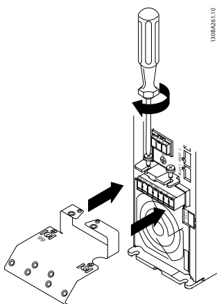
Illustration 6.2 Installation de la plaque de montage
