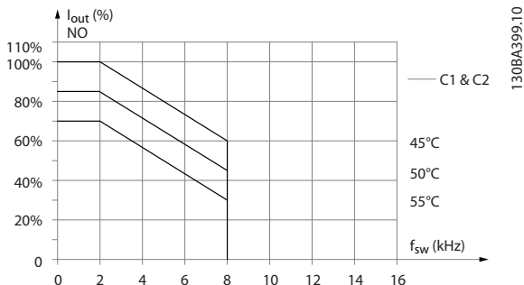
Illustration 9.18 Déclassement de I sortie pour différentes T AMB , MAX pour protections de types C1 et C2, utilisant SFAVM en mode surcharge normale (surcouple de 110 %)
