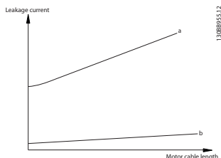
Illustration 2.35 Influence de la longueur de câble et de la puissance sur le courant de fuite. Pa > Pb
