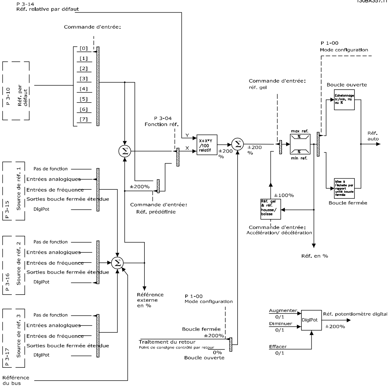
Illustration 2.29 Schéma du bloc présentant la référence distante
