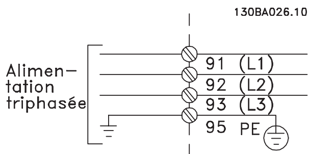
Illustration 6.1 Mise sous tension
