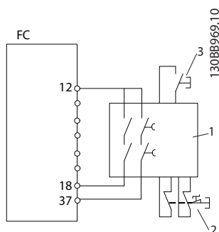
Illustration 2.4 Exemple SS1
