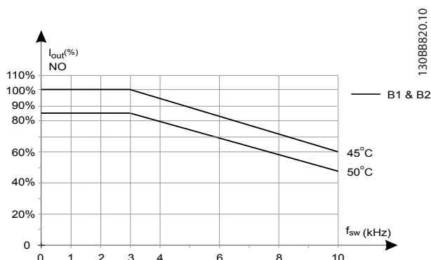
Illustration 9.12 Déclassement du courant de sortie avec fréquence de commutation et température ambiante pour variateurs de fréquence de 600 V, protection de type B, 60° AVM, NO
