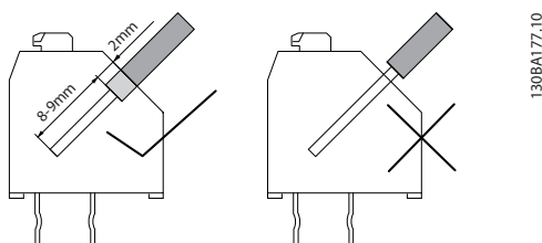
Ilustración 3.8 Montaje
