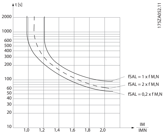
Ilustración 2.40 El eje X muestra la relación entre los valores I_{motor} e I_{motor\ nominal} . El eje Y muestra el intervalo en segundos que transcurre antes de que el ETR se corte y desconecte el convertidor de frecuencia. Las curvas muestran la velocidad nominal característica al doble de la velocidad nominal y al 0,2x de la velocidad nominal.
