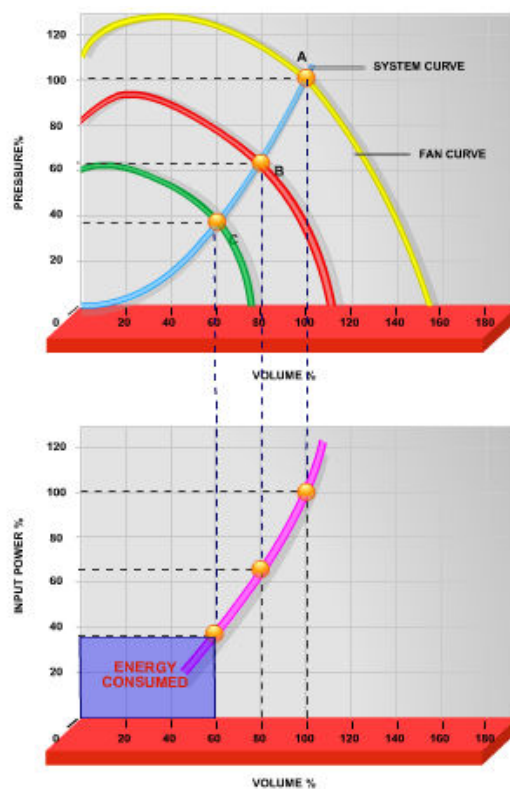
Ilustración 2.9 Cuando se utiliza un convertidor de frecuencia para reducir la capacidad del ventilador al 60 %, es posible obtener un ahorro energético de más del 50 % en equipos convencionales.
