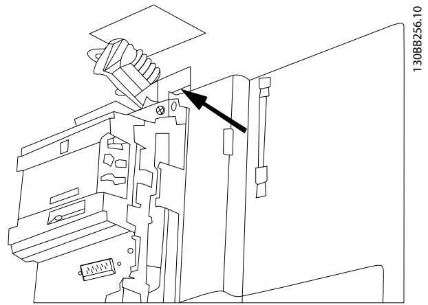
Ilustración 6.47 Conexión superior para bus de campo en unidades NEMA 1
