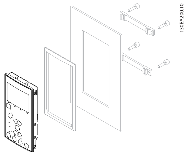
Ilustración 3.17 Kit LCP con LCP numérico, sujeciones y junta.
