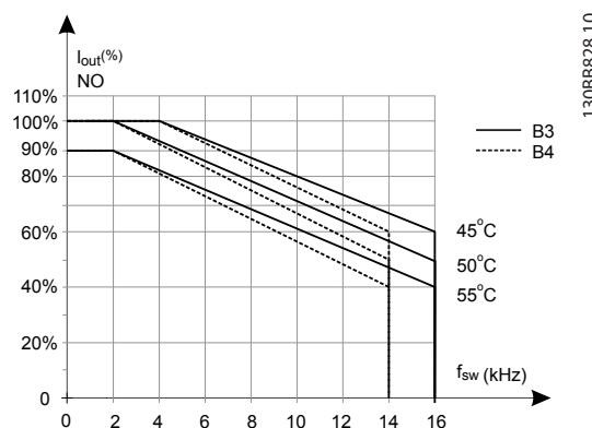
Ilustración 9.9 Reducción de potencia de I_{out} para diferentes T_{AMB, MÁX.} para tipos de protección B3 y B4, utilizando AVM de 60° en modo de sobrecarga normal (110 % por encima del par)
