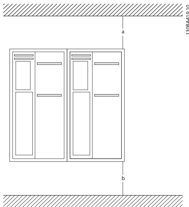
Ilustración 5.2 Separación
