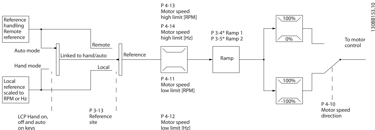
Ilustración 2.24 Estructura de lazo abierto
