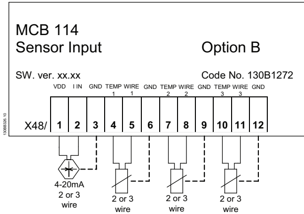
Ilustración 3.15 Cableado eléctrico
