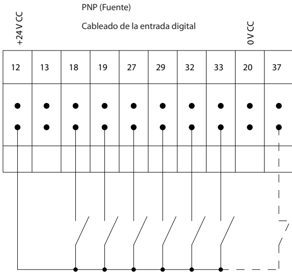
Ilustración 6.56 Polaridad de entrada PNP (fuente)
