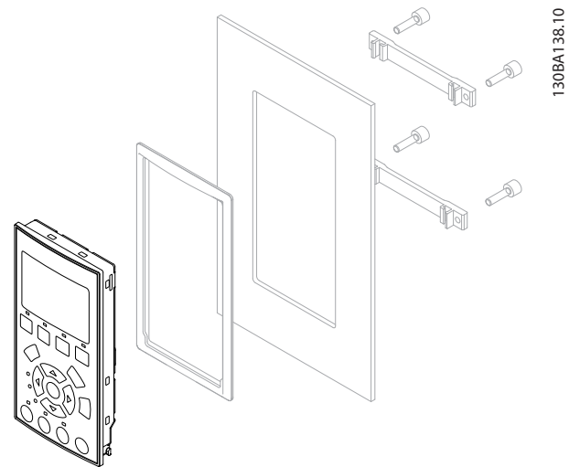
Ilustración 3.16 Kit LCP con LCP gráfico, sujeciones, cable de 3 m y junta.
