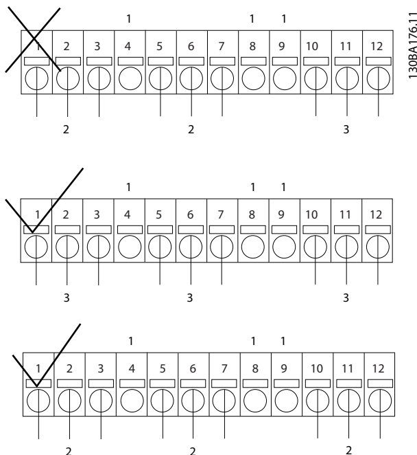
Ilustración 3.9 Conexión
