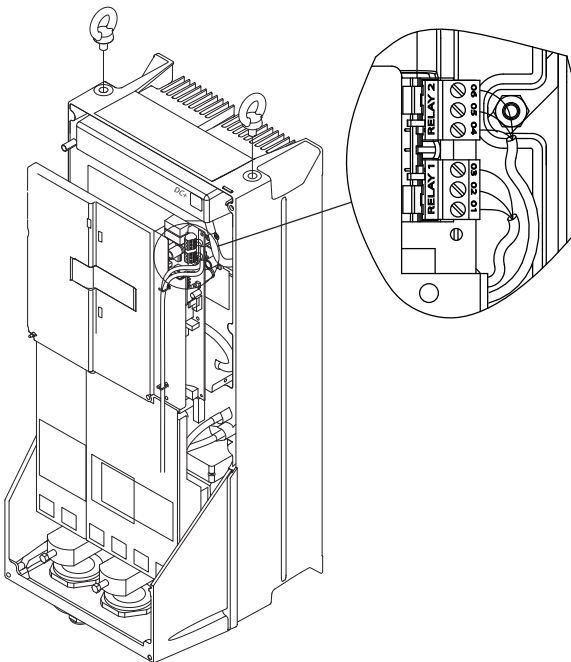
Afbeelding 6.37 Klemmen voor relaisaansluiting (behuizingstype C1 en C2)
