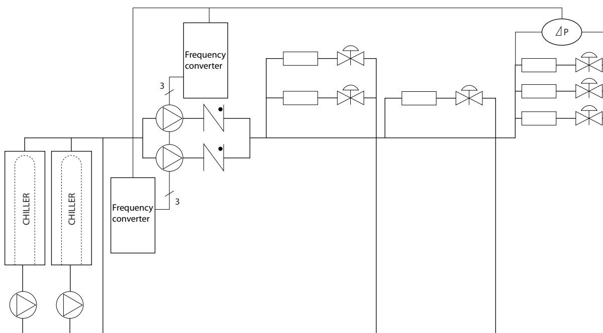
Afbeelding 2.22 De VLT-oplossing
