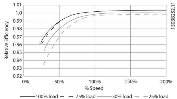
Afbeelding 9.2 Typische rendementscurves
