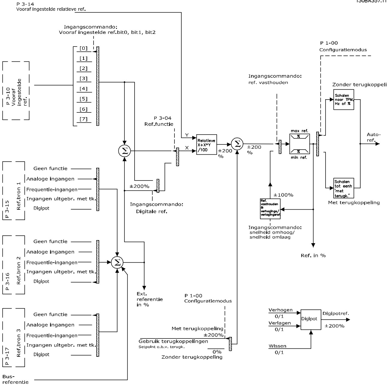
Abbeelding 2.29 Blokschema voor externe referentie
