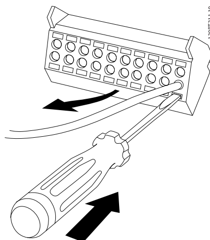
Afbeelding 6.52 Kabel insteken
