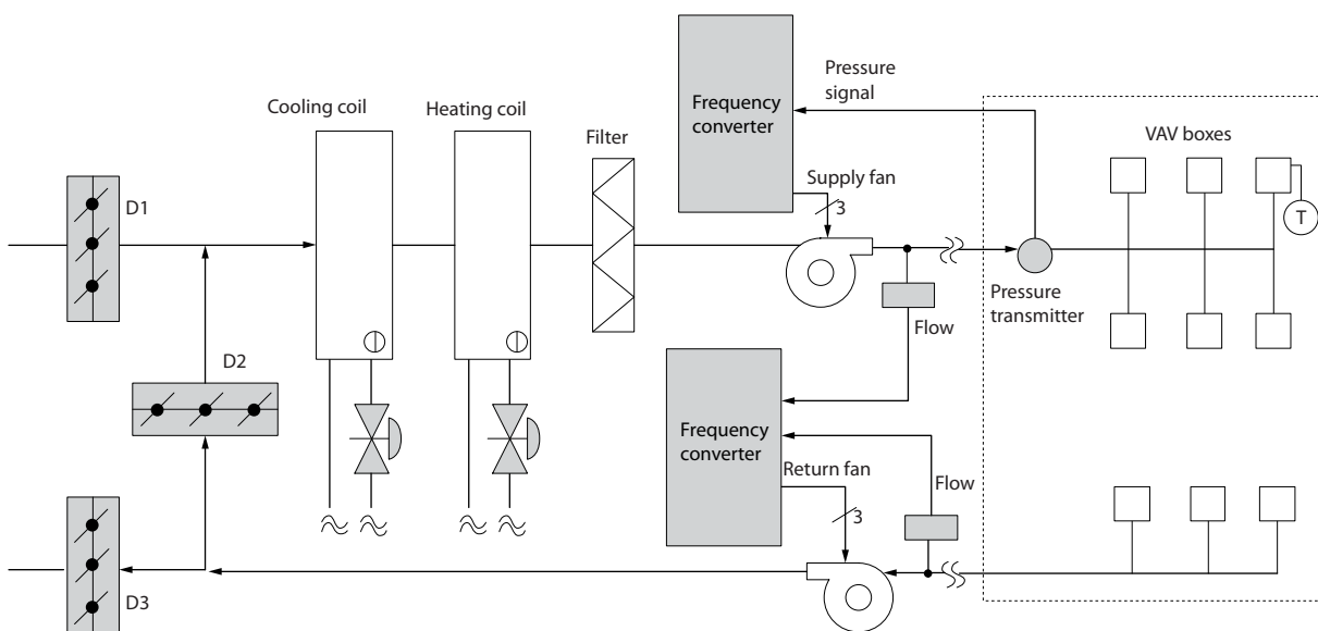
Afbeelding 2.17 De VLT-oplossing
