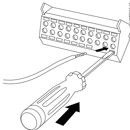
Afbeelding 6.51 Schroevendraaier insteken
