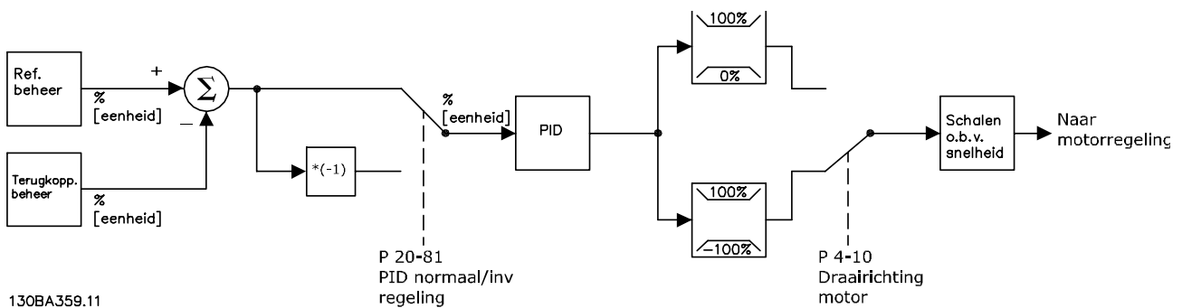
Afbeelding 2.26 Blokschema van de terugkoppelsregelaar
