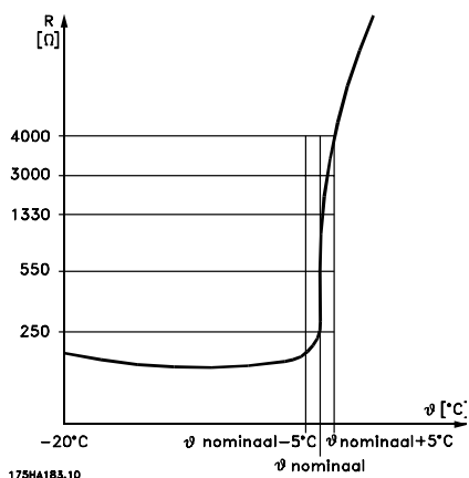
Afbeelding 2.41 Uitschakeling van de thermistor
