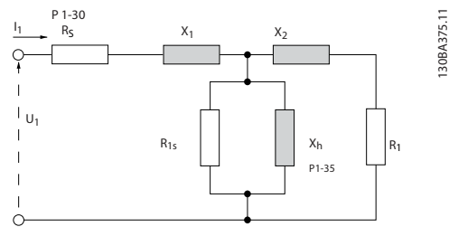
Рисунок 3.4 Эквивалентная схема асинхронного двигателя
