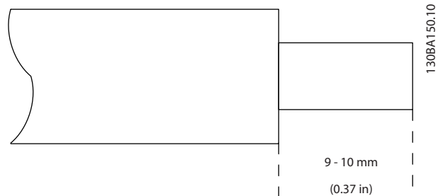
Abbildung 4.17 Abisolieren
