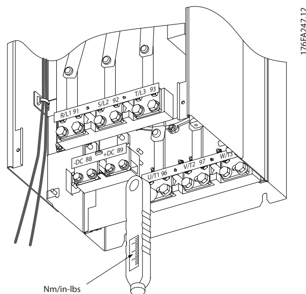
Abbildung 4.10 Festziehen der Schrauben mit einem Drehmomentschlüssel
