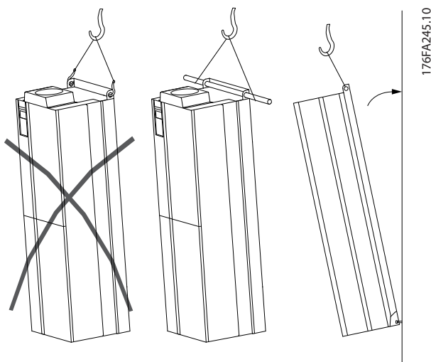
Abbildung 3.2 Empfohlenes Hebeverfahren, Baugröße E
