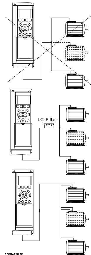
Abbildung 4.32 Parallel Motoranschluss
