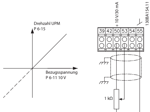
Abbildung 4.30 Potenziometer-Sollwert
