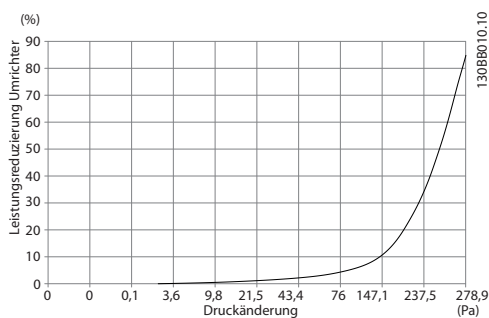
Abbildung 3.31 Baugröße E Leistungsreduzierung vs. Druckänderung (kleiner Lüfter), P315T4 und P450T7-P500T7 Luftzirkulation des Frequenzumrichters: 650 cfm (1105 m³/h)
