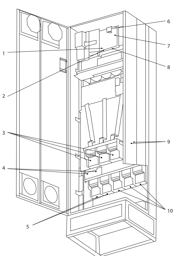
Abbildung 4.3 Kompaktformat IP21 (NEMA 1) und IP54 (NEMA 12) Gehäusetyp E1
