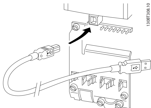
Abbildung 5.14 USB-Anschluss am Frequenzumrichter
