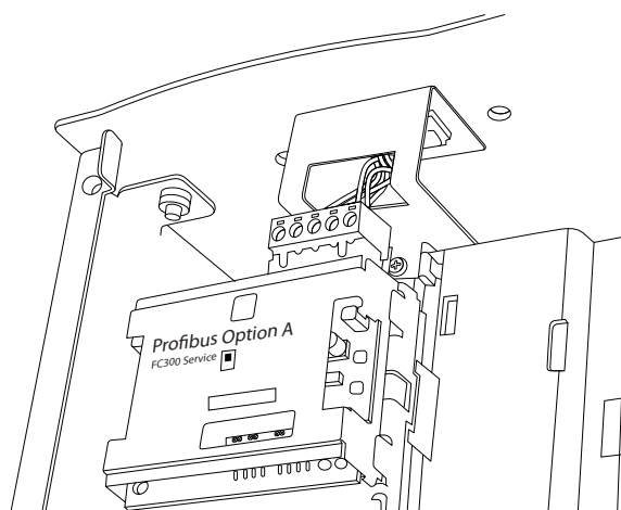
Abbildung 4.14 Oberer Eingang der Feldbuskabel.
