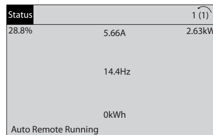
Εικόνα 6.2 Βήμα 1: Ενεργοποιήστε το μετατροπέα συχνότητας (κίτρινες λυχνίες LED)
