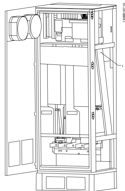
Εικόνα 4.14 Διαδρομή καλωδίωσης κάρτας ελέγχου για F1/F3. Διαδρομή καλωδίωσης κάρτας ελέγχου για F2/F4 Χρησιμοποιήστε την ίδια διαδρομή
