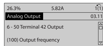
Рисунок 6.7 Выбран параметр Параметр 6-50 Клемма 42, выход
