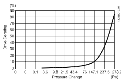
Afbeelding 3.12: Reductie frame E t.o.v. drukverandering (kleine ventilator), P250T5 en P355T7-P400T7
