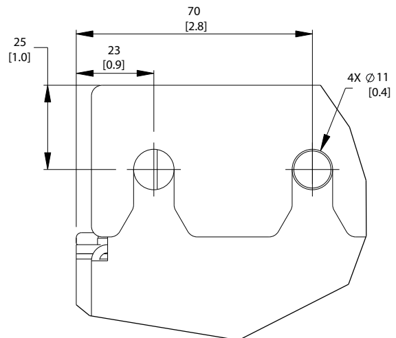
Рисунок 5.16 Детальный чертеж верхнего монтажного отверстия, D8h
