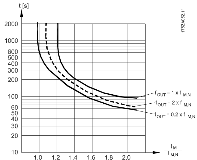
Рисунок 5.1 Характеристики ЭТР
