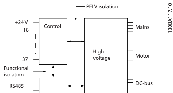
Рисунок 7.1 Изоляция PELV
