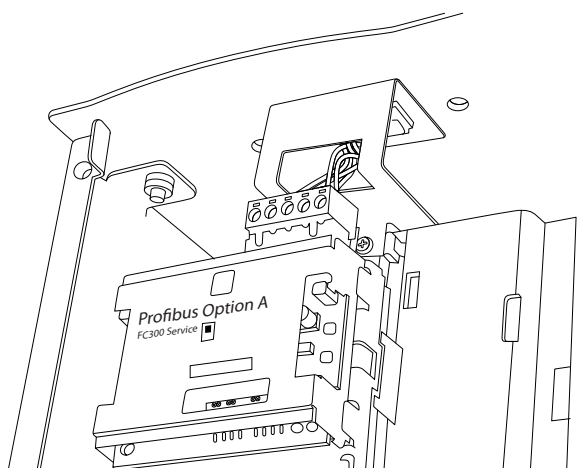
Рисунок 10.10 Подключение периферийной шины сверху
