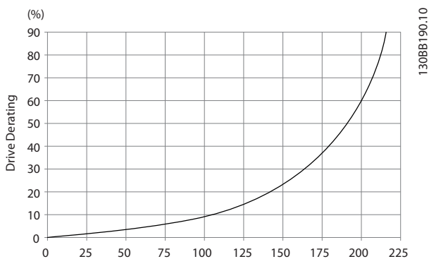
Рисунок 9.7 Снижение номинальных характеристик в зависимости от изменения давления для корпусов F1–F4. Циркуляция воздуха: 580 куб. футов/мин (985 м 3 /ч)
