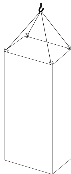
Рисунок 9.4 Рекомендуемый способ подъема для корпусов F8
