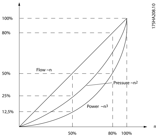
Рисунок 5.9 Законы пропорциональности
