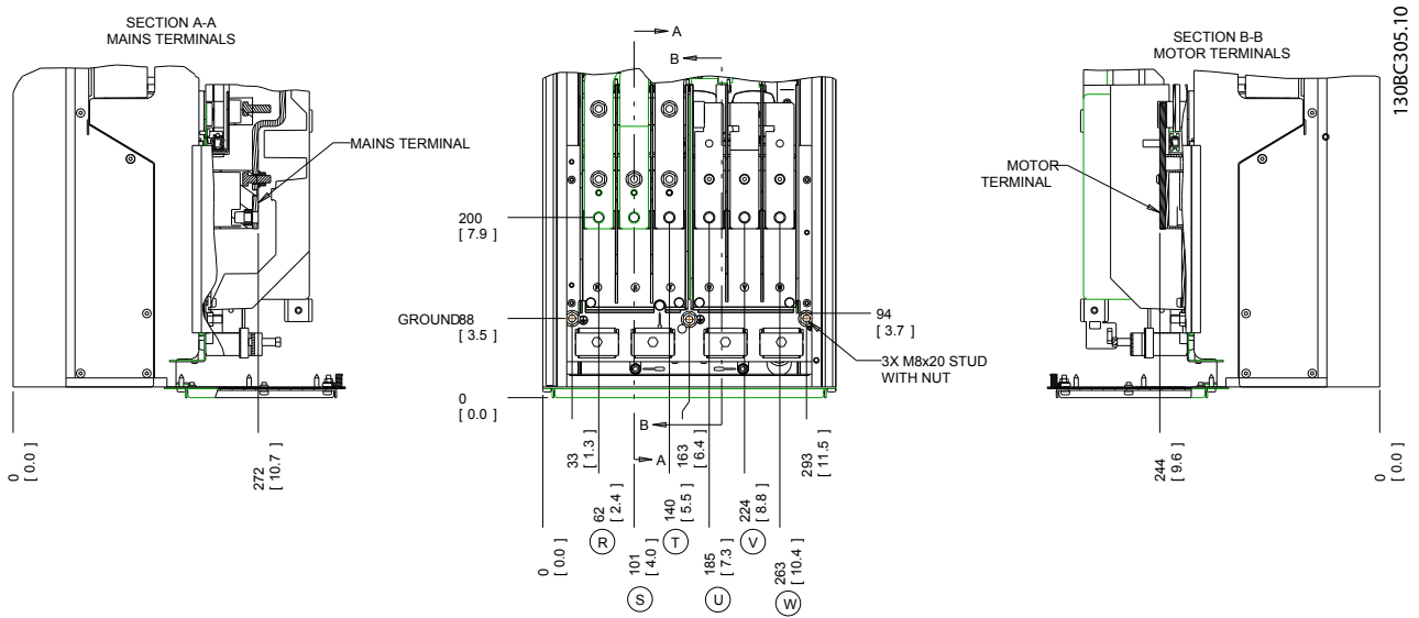
Slika 2.7 Lokacije stezaljki D1h
