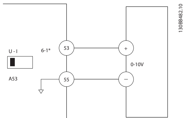
Slika 5.10 Primjer ožičenja za vanjski uređaj koji daje upravljački signal 0-10 V
