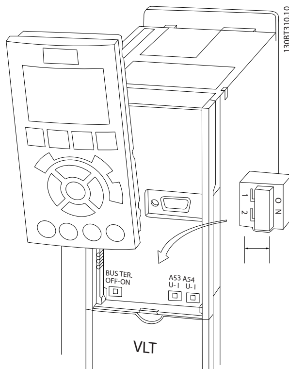
Slika 2.31 Lokacija sklopki stezaljke 53 i 54 i sklopke zaključenja sabirnice
