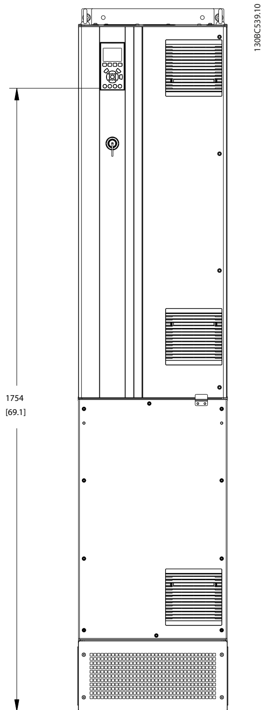
Slika 1.3 Kućište D7h
