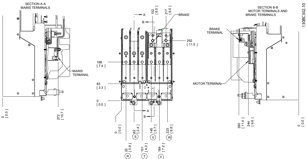
Slika 2.8 Lokacije stezaljki D3h
