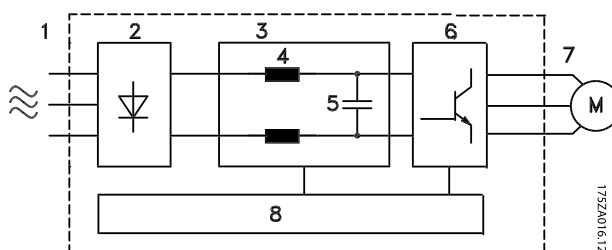
图 1.4 变频器框图
