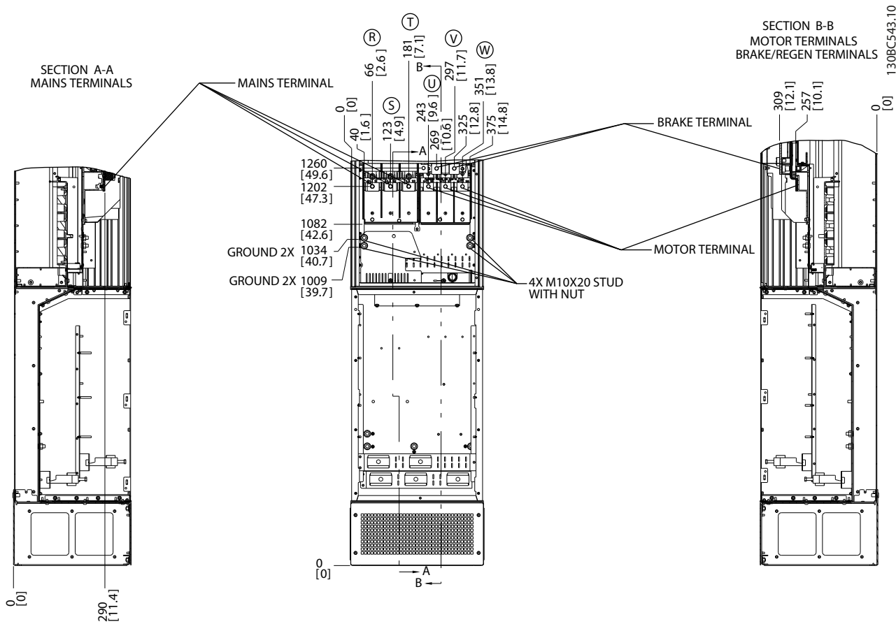
图 2.19 端子位置, D7h (配备制动选件)
