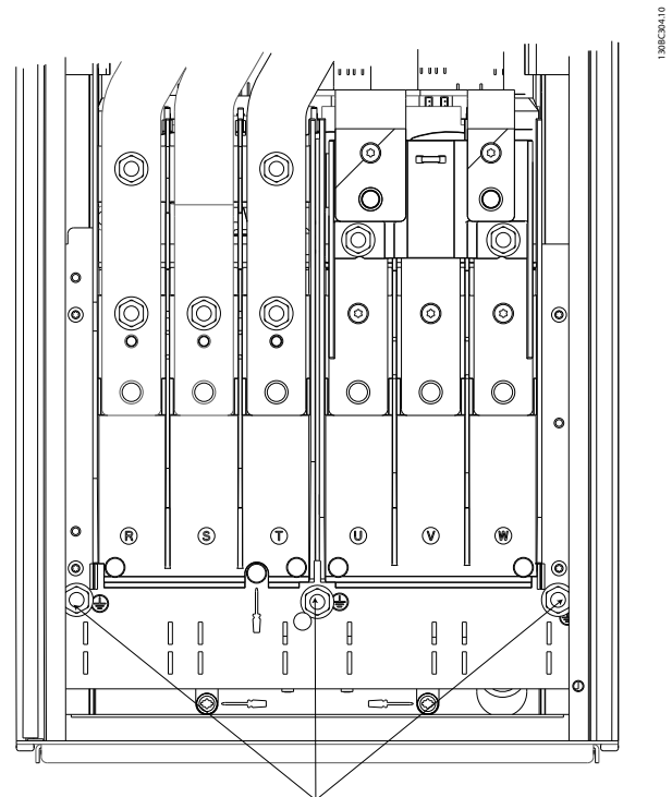
图 2.6 IP21/54 机箱的接地
