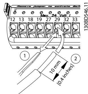
图 4.26 连接控制线缆
