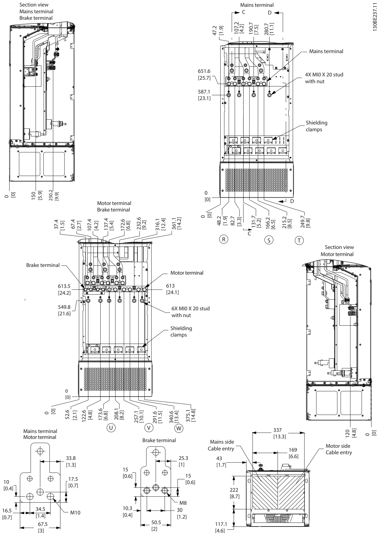
图 4.19 超大配线柜 — D7h
