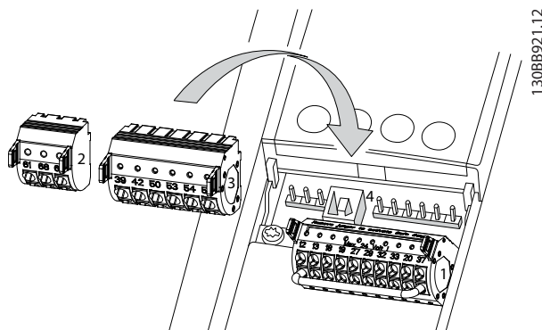
图 4.24 控制端子位置
