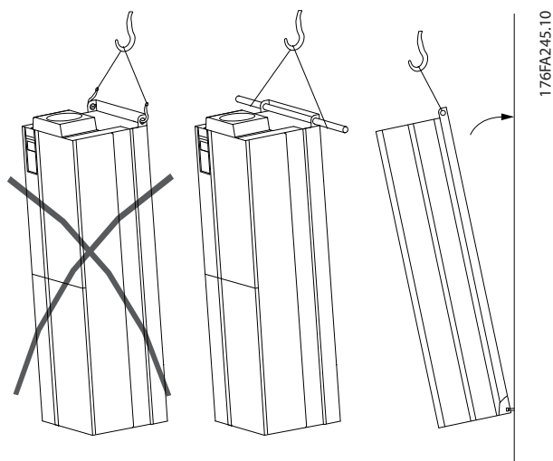
图 3.2 建议的起吊方法
