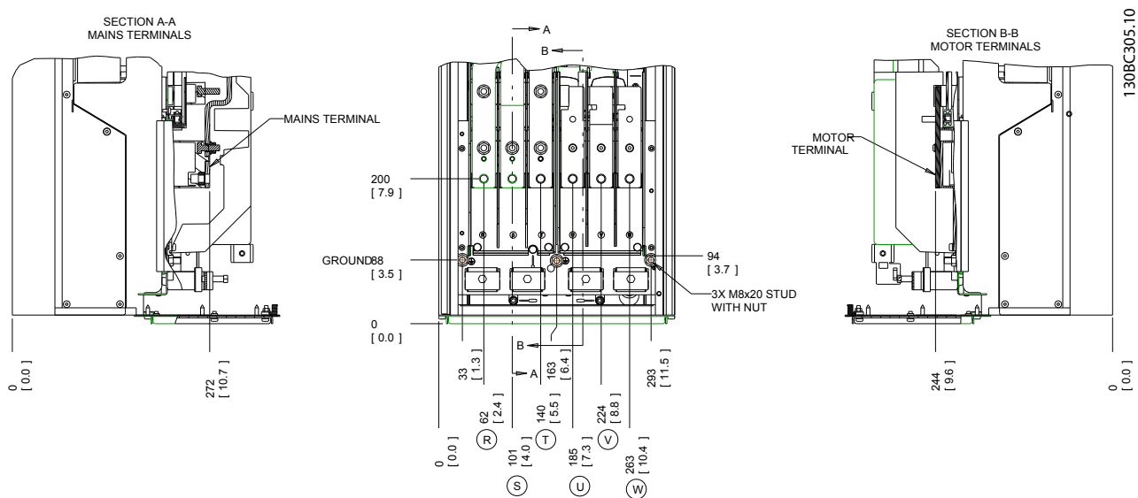
图 4.5 端子位置 — D1h
