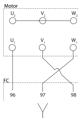
Slika 5.5 Ožičenje za promenu smera motora
