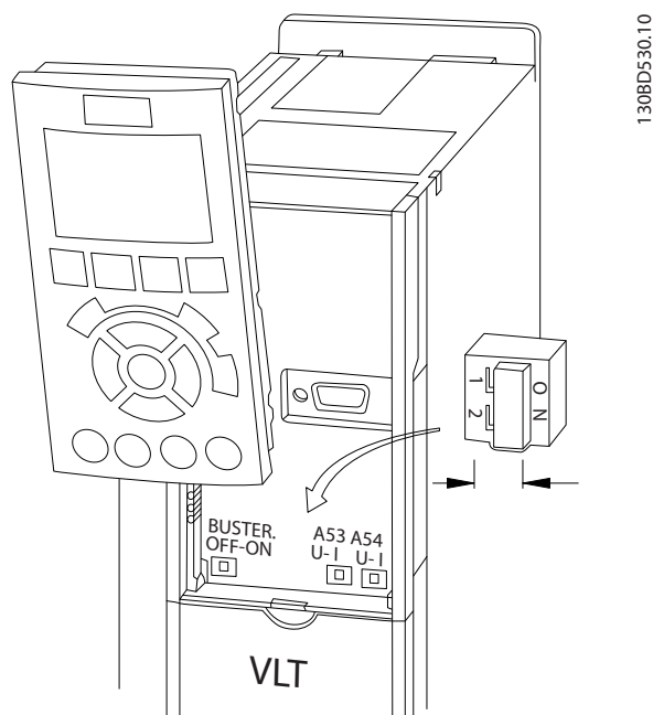
Slika 4.27 Lokacija prekidača priključaka 53 i 54
