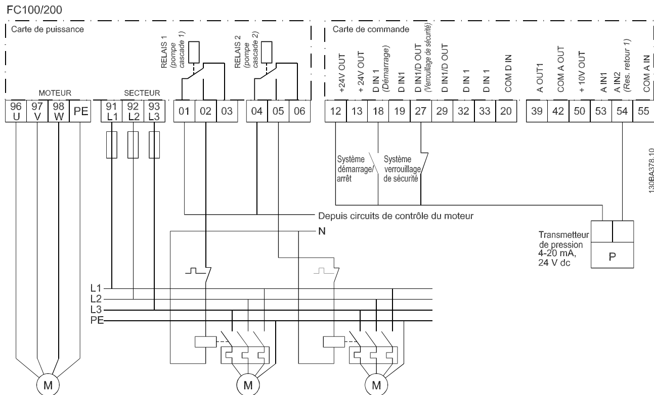
Illustration 8.4 Schéma de câblage du contrôleur de cascade
