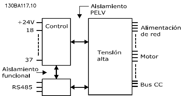
Ilustración 10.1 Aislamiento PELV
