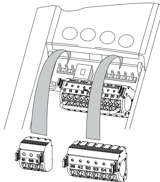
Ilustración 5.35 Ubicaciones de los terminales de control
