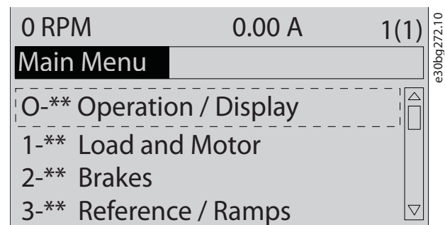
Kuva 3.7 Päävalikkonäkymä
