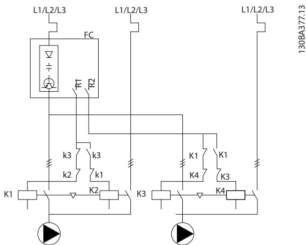
Εικόνα 8.6 Διάγραμμα καλωδίωσης εναλλαγής οδηγήτριας αντλίας
