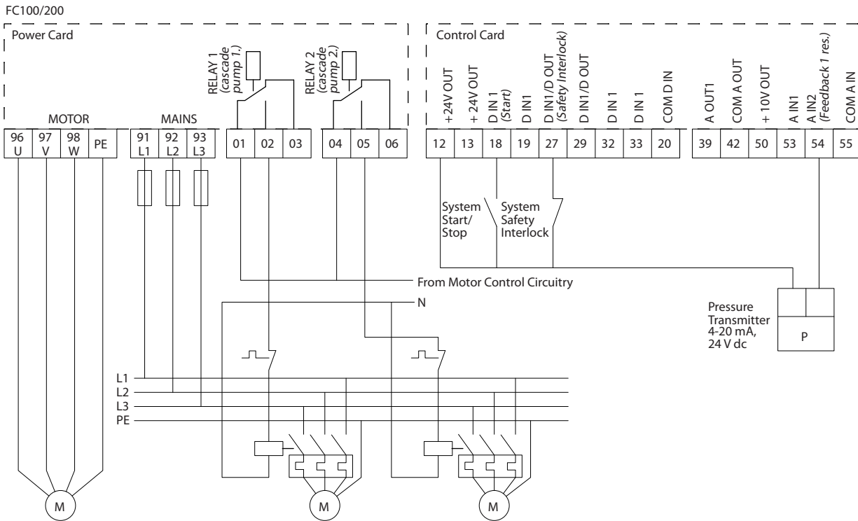
Εικόνα 8.4 Διάγραμμα καλωδίωσης ελεγκτή διαδοχικών βαθμίδων
