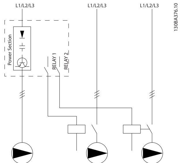
Εικόνα 8.5 Διάγραμμα καλωδίωσης για σταθερή αντλία μεταβαλλόμενης ταχύτητας
