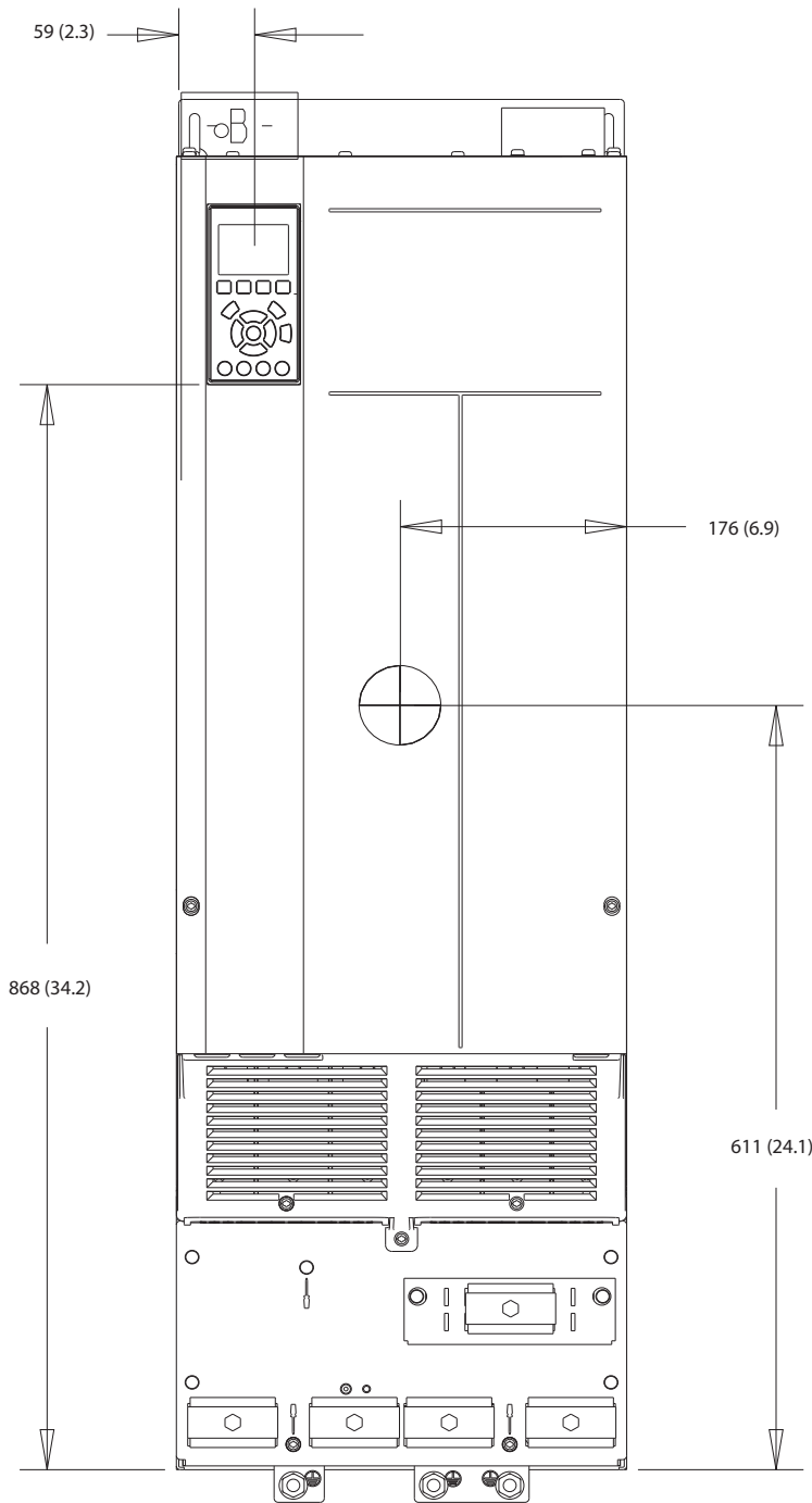
Εικόνα 10.15 Μπροστινή όψη του D4h
