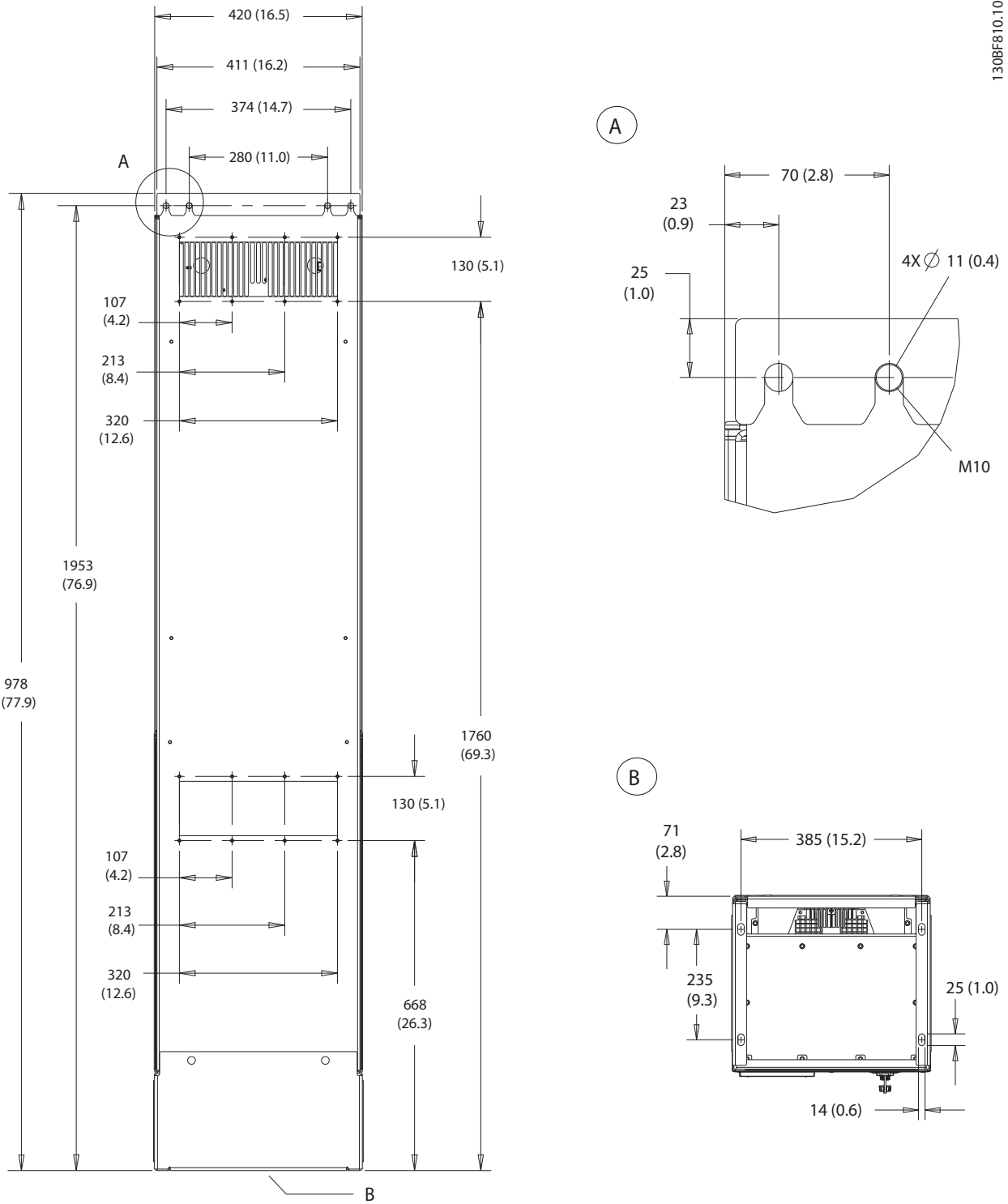
图 10.32 D7h 的后视图
