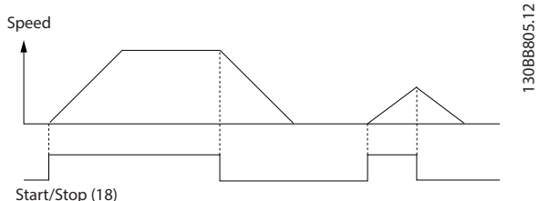
图 8.1 带 Safe Torque Off 的启动/停止
