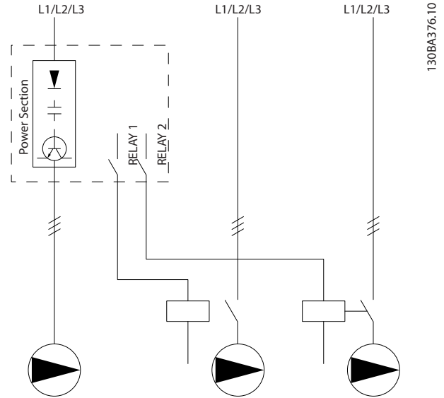
Çizim 8.5 Sabit Değişken Hız Pompası Kablo Tesiatı Şeması
