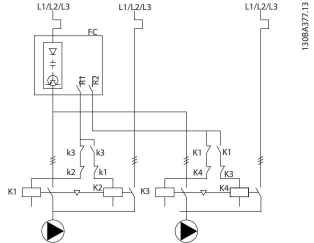
Çizim 8.6 Birinci Pompa Alternasyonu Kablo Tesiatı Şeması
