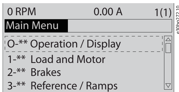
Obrázek 3.7 Hlavní menu
