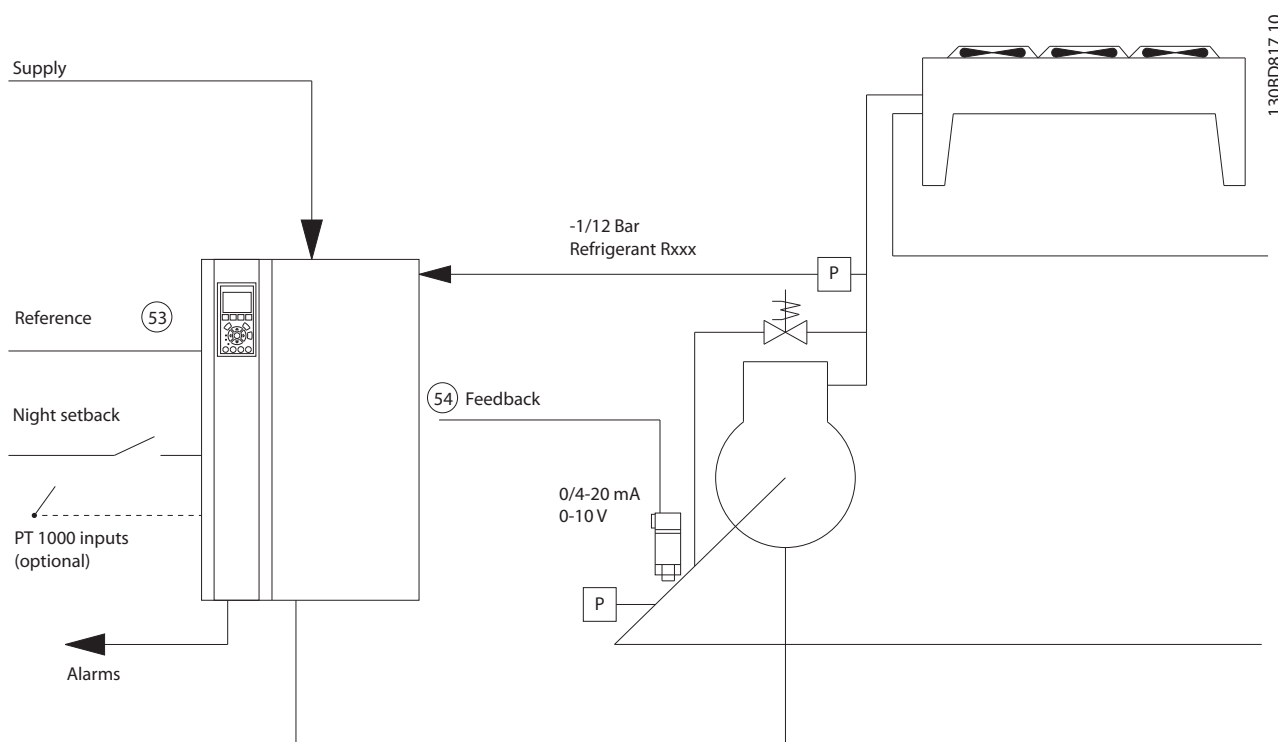
Abbildung 6.1 Standardzeichnung eines „Verdichters mit interner Regelung“
