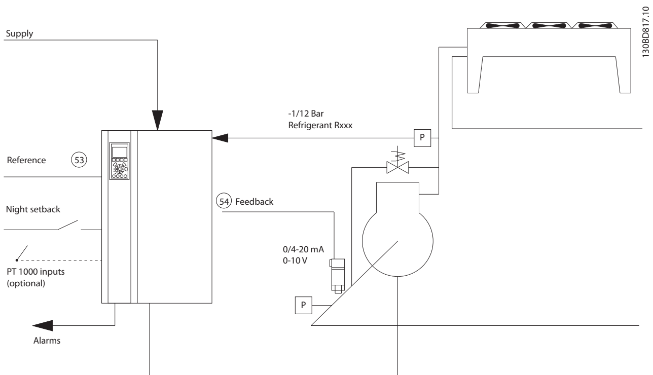
Εικόνα 6.1 Τυπικό σχέδιο "Συμπιεστή με εσωτερικό έλεγχο"
