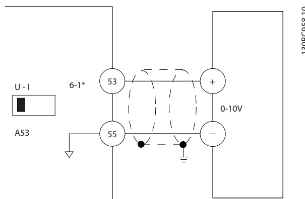
Illustration 6.8 Exemple de câblage d'un dispositif externe fournissant un signal de commande 0-10 V (variateur de fréquence à gauche, dispositif externe à droite)
