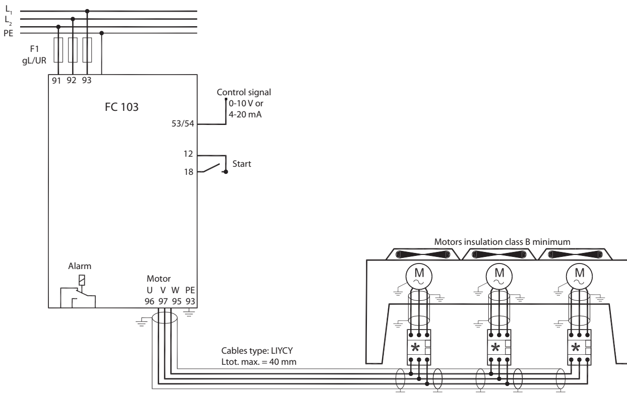
Illustration 7.2 Commande de vitesse utilisant la référence analogique (boucle ouverte) – ventilateur ou pompe unique/ventilateurs ou pompes multiples en parallèle
