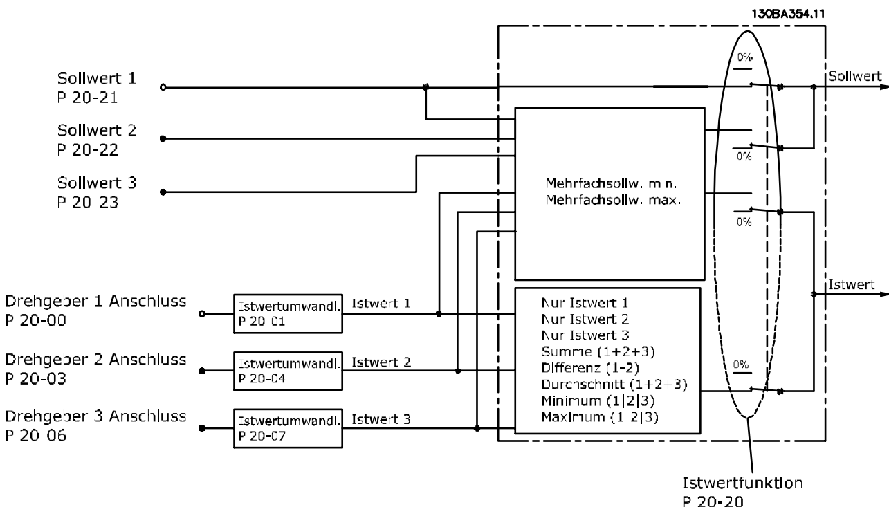
Abbildung 3.46 Istwert
