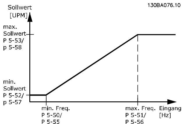
Abbildung 3.28 Pulseingang
