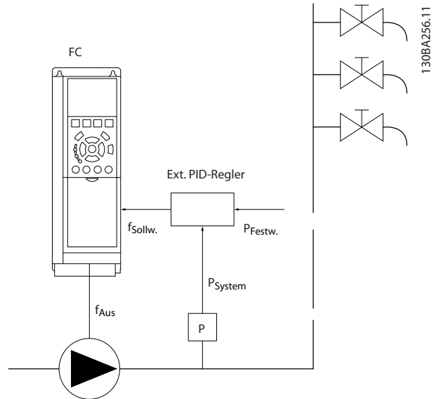
Abbildung 3.52 Boost-System
