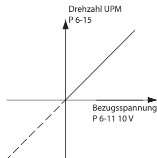
Abbildung 1.9 Potenziometer Sollwert
