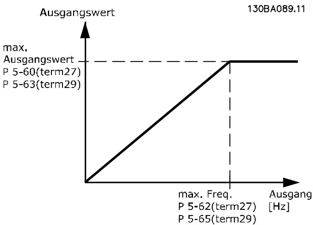
Abbildung 3.29 Pulsausgänge
