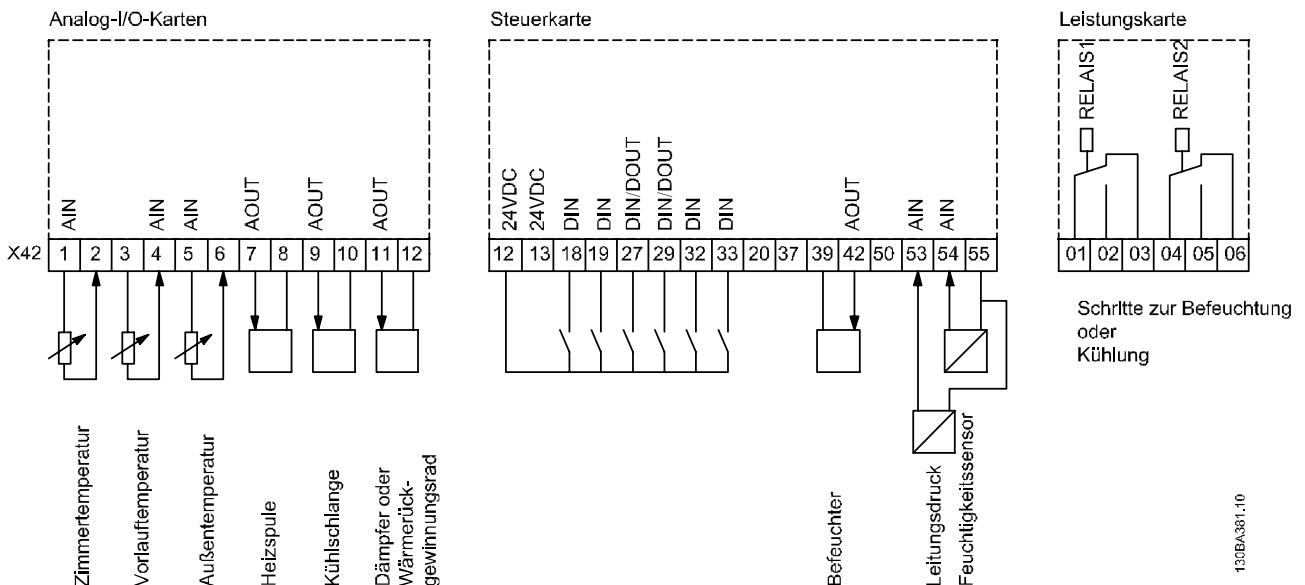
Abbildung 3.69 Analog-E/A-Option MCB 109
