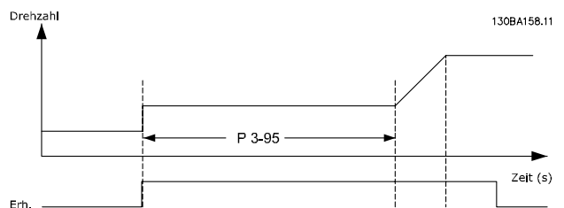
Abbildung 3.22 Rampenverzögerung Fall 1
