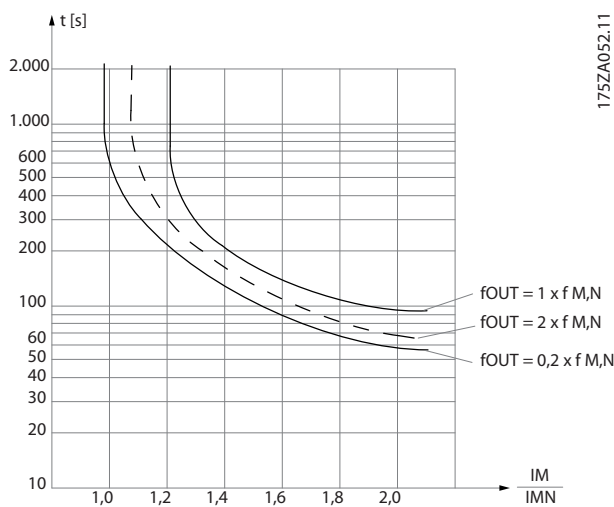
Abbildung 3.14 ETR-Profil
