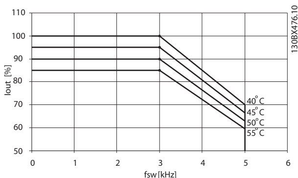
Ilustração 8.2 Derating do gabinete metálico tamanho D, N160 a N250 380–480 V (T5) Sobrecarga normal de 110%, SFAVM
