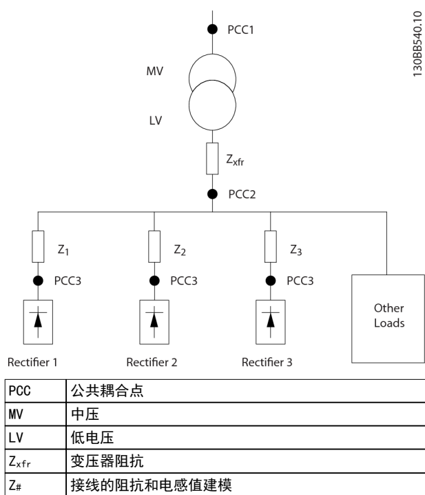
图 1.10 小配电系统
