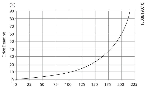
图 3.4 F 机箱的降额与 降容
