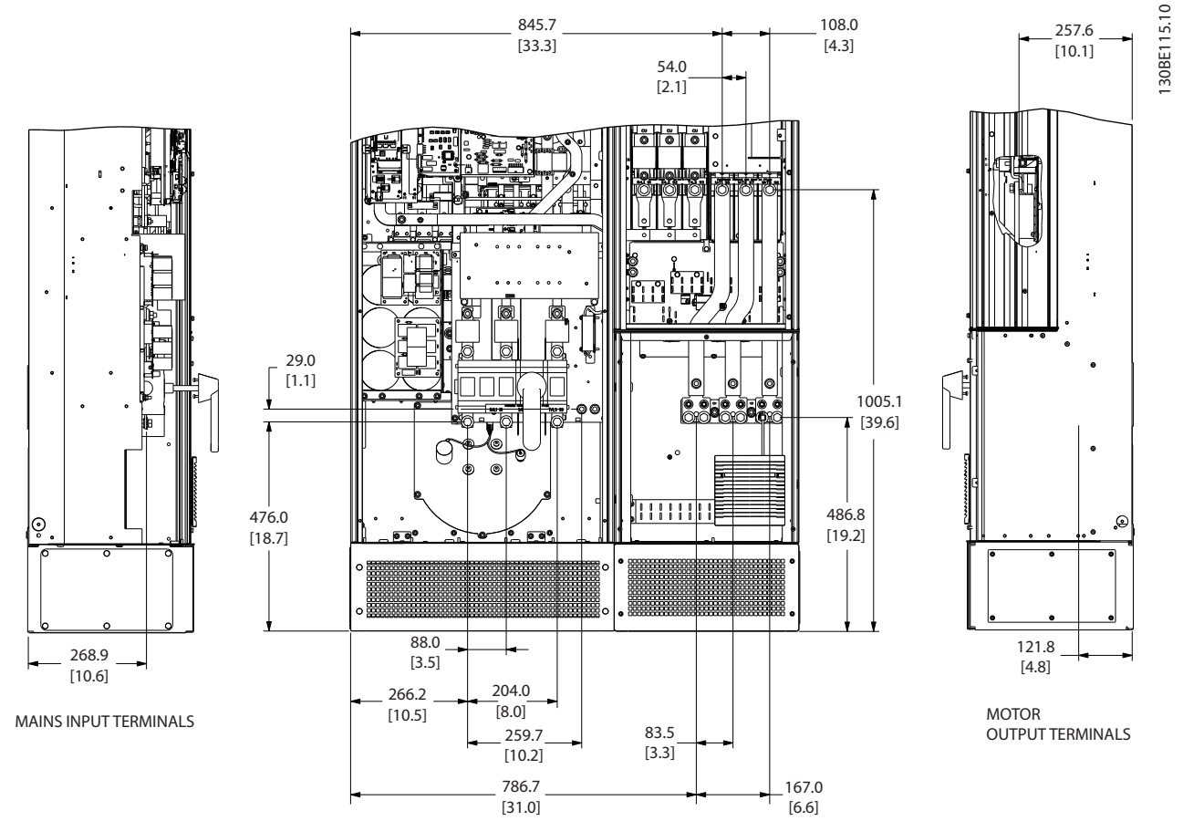
图 3.13 端子位置, 机箱规格 D2n
