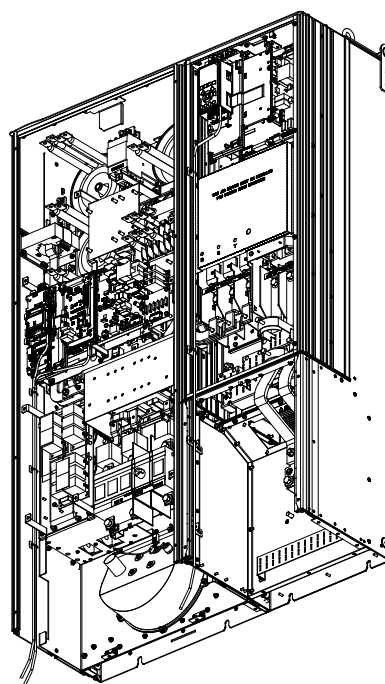
图 4.6 机箱规格 D2n 的控制卡接线路径
