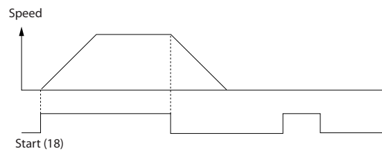
图 6.2 带 Safe Torque Off 选项的启动/停止命令
