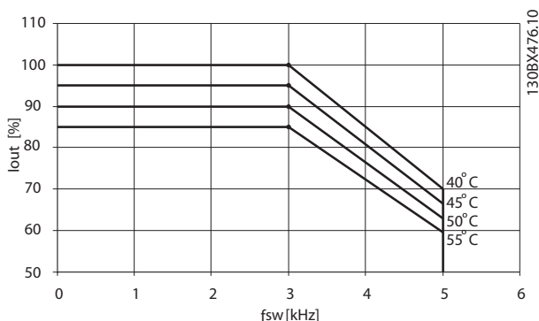
图 8.2 降容曲线 - 机箱规格 D、N160 至 N250 380-480 V (T5) 正常过载 110%、SFAWM
