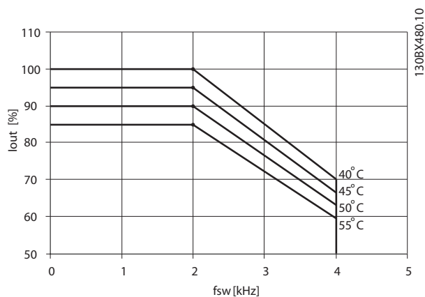
图 8.4 降容曲线 - 机箱规格 E 和 F、P315 至 P710 380-480 V (T5) 正常过载 110%、SFAWM
