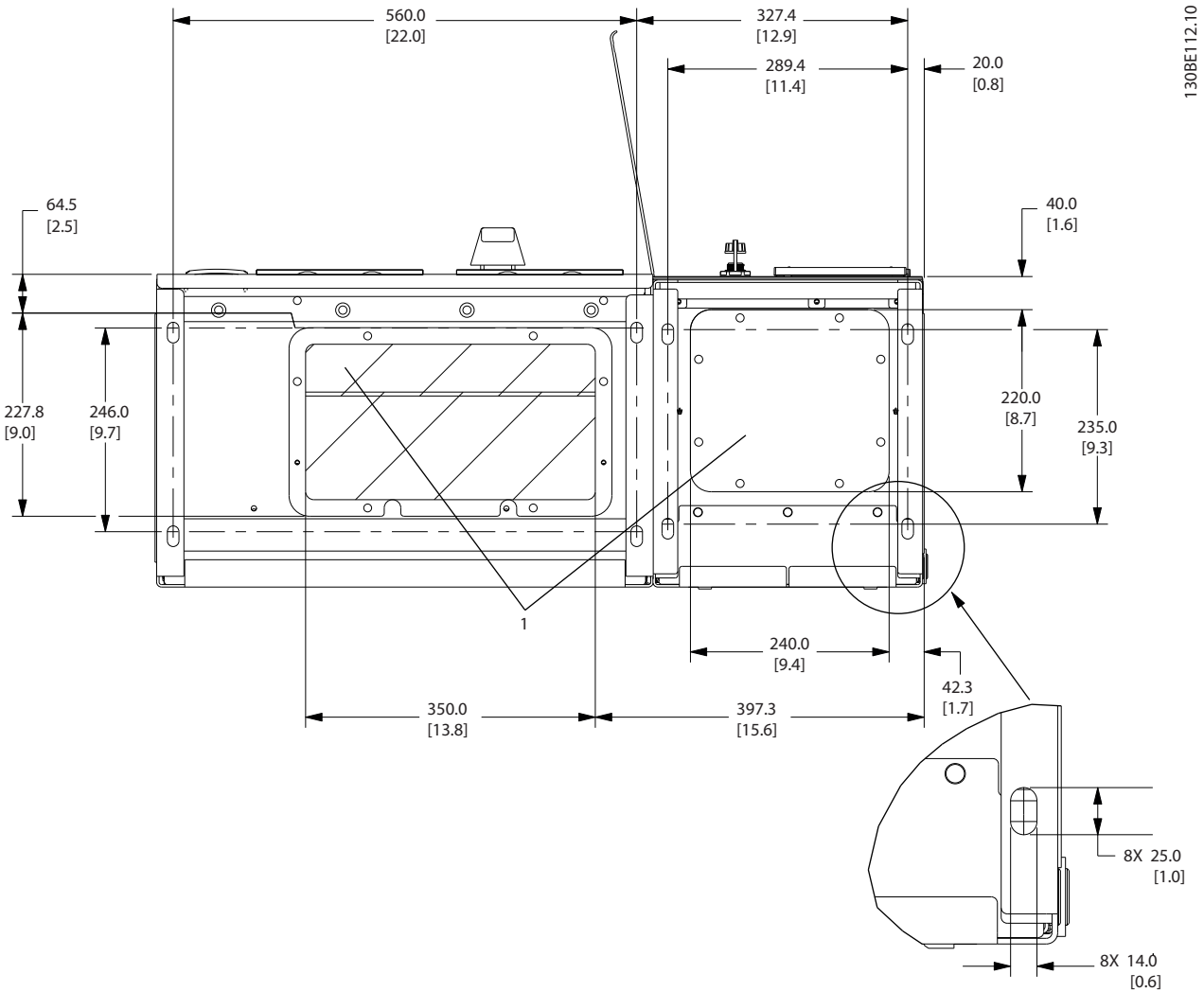
底视图, D1n/D2n
