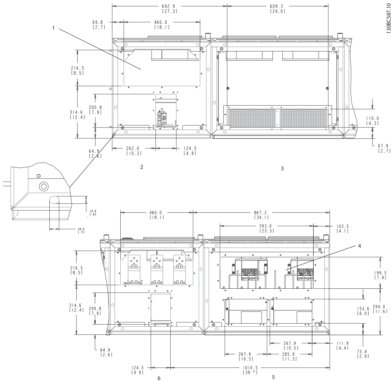
底视图, F18
