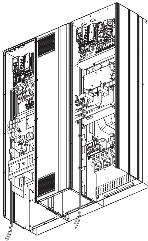
图 4.7 机箱规格 E9 的控制卡接线路径
