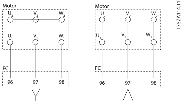
图 4.2 Y 形和三角形端子配置
