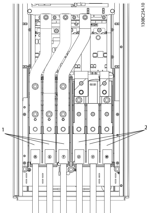
圖 2.13 連接至交流電主電源
