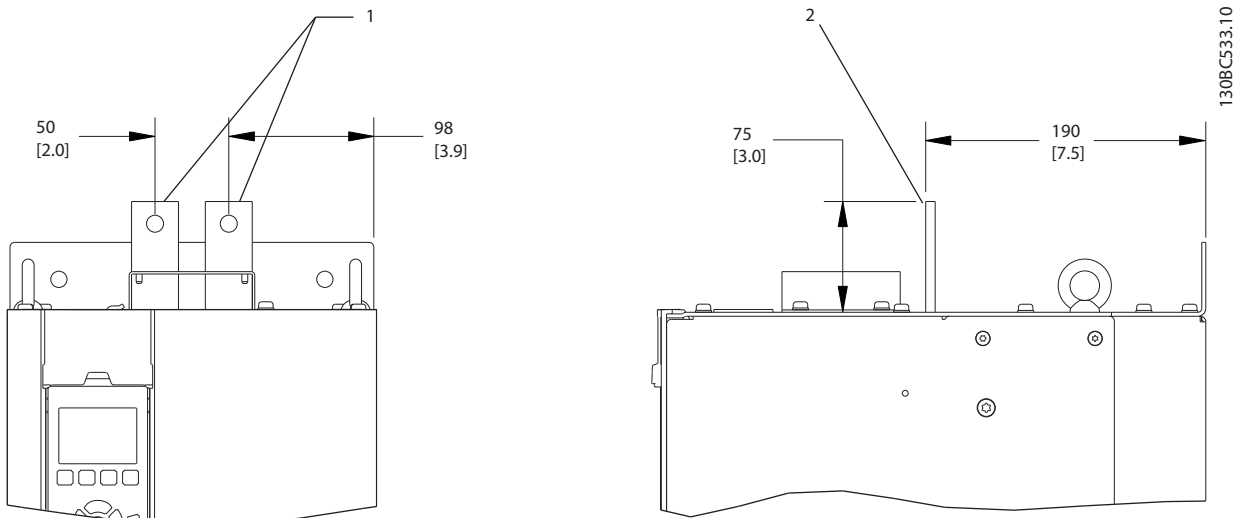
圖 2.9 負載共償或再生端子, D3h
