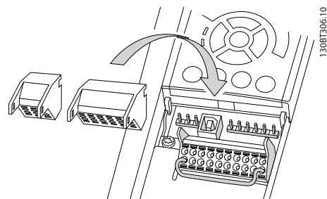
圖 2.20 移除控制端子
