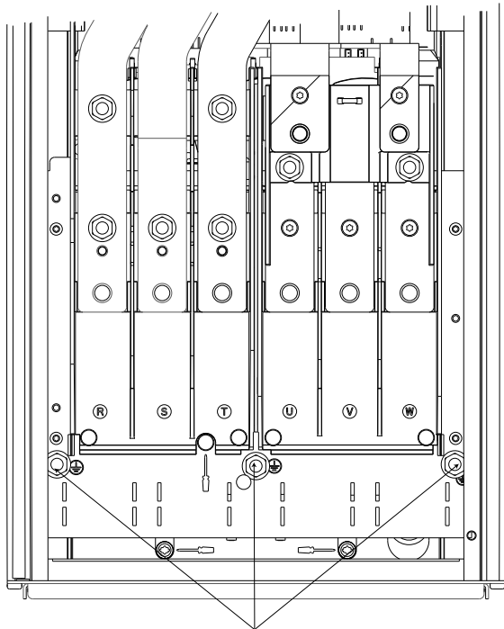
圖 2.6 IP21/54 外殼的接地
