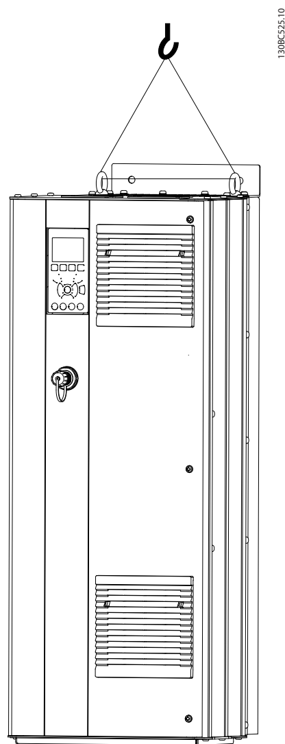
圖 2.1 建議的吊掛方式
