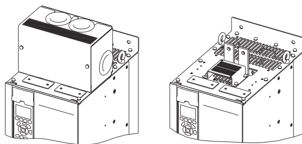
圖 2.22 含蓋 (L) 和未含蓋 (R) 的負載共償或再生端子
