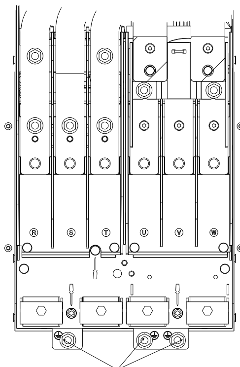
圖 2.5 IP20 (底架) 外殼的接地點
