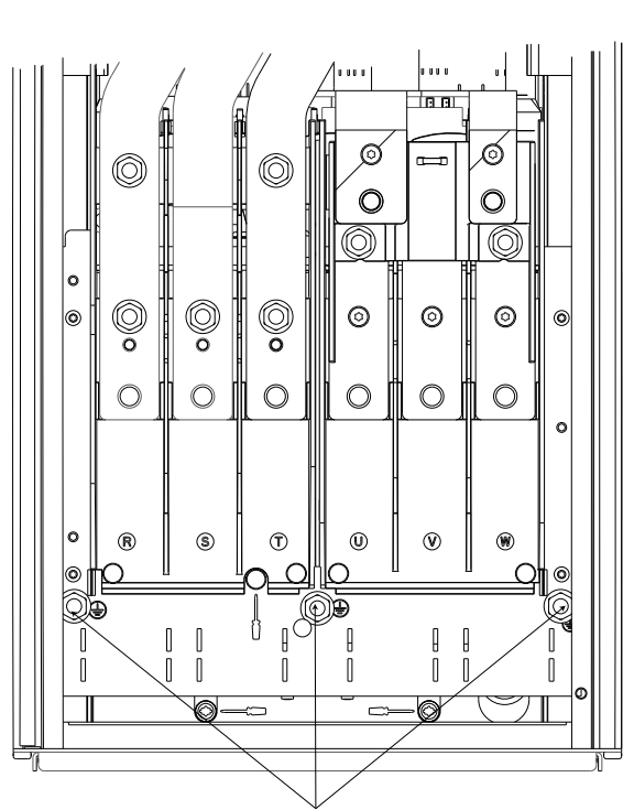
Рисунок 2.6 Заземление (зануление) для корпусов IP21/54.
