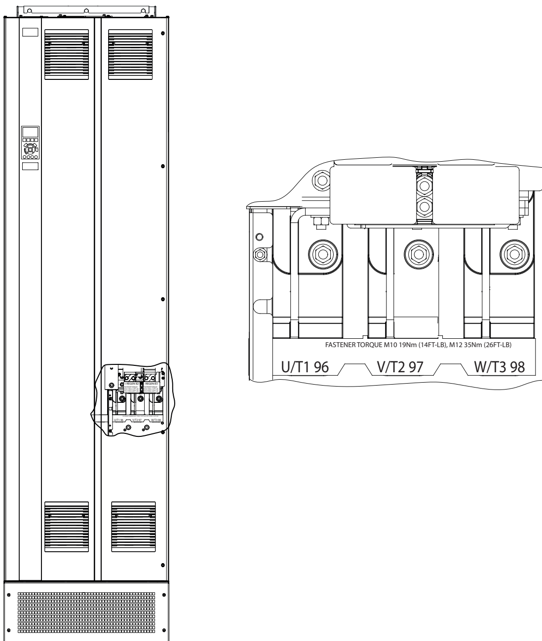
Illustration 5.3 Bornes de moteur CA (boîtier E1h indiqué). Pour une vue détaillée des bornes, se reporter au chapitre 5.7 Dimensions des bornes .
