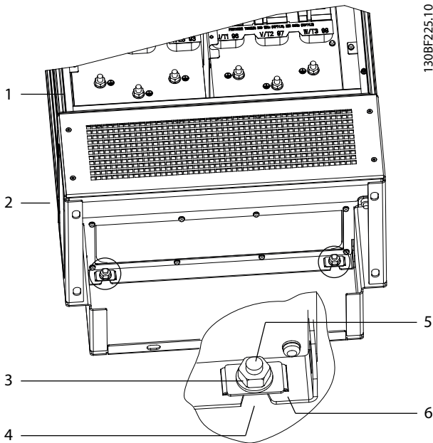
Illustration 4.5 Points de fixation du socle au boîtier
