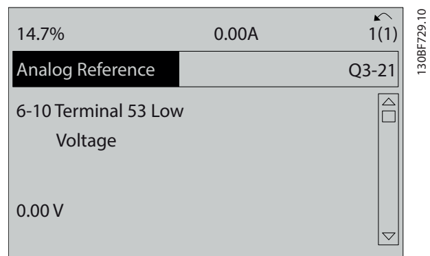
Illustration 6.8 Paramètre 6-10 Ech.min.U/born.53
