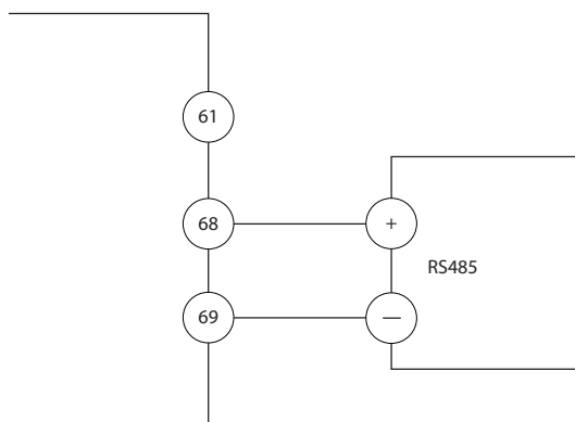
Illustration 5.21 Schéma de câblage de la communication série
