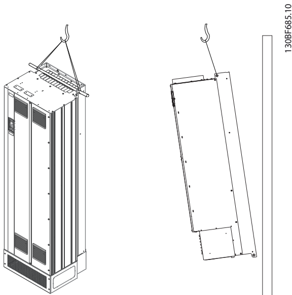
Illustration 4.2 Méthode de levage recommandée
