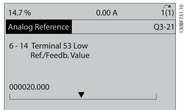
Illustration 6.10 Paramètre 6-14 Val.ret./Réf.bas.born.53
