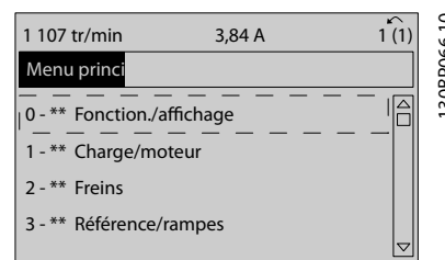
Illustration 6.2 Affichage du menu principal
