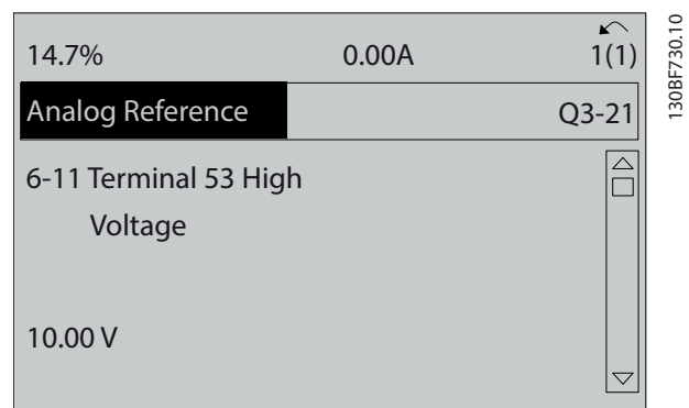
Illustration 6.9 Paramètre 6-11 Ech.max.U/born.53
