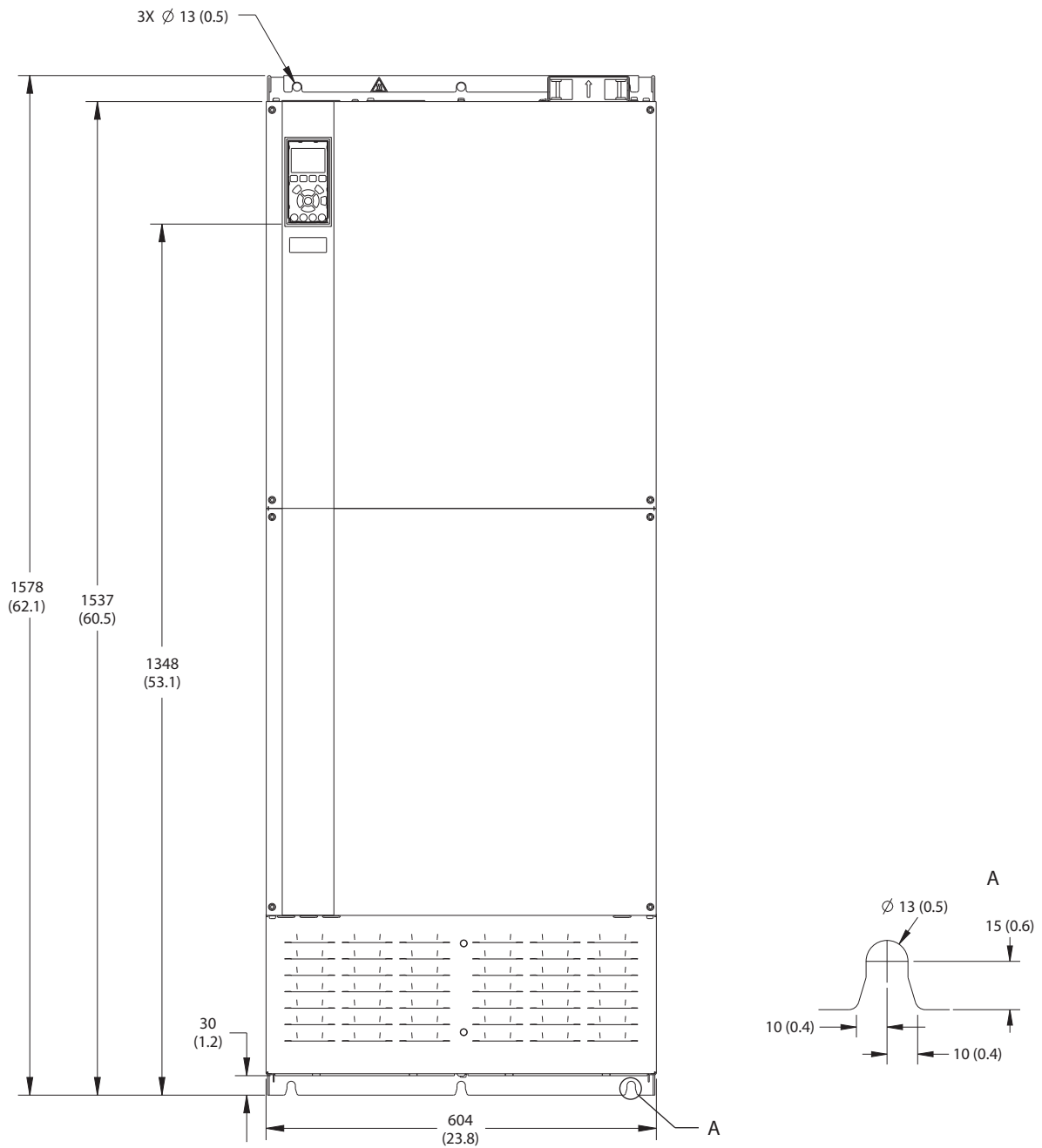
Illustration 9.14 Vue frontale du boîtier E4h
