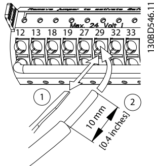
Illustration 5.20 Raccordement du câblage de commande
