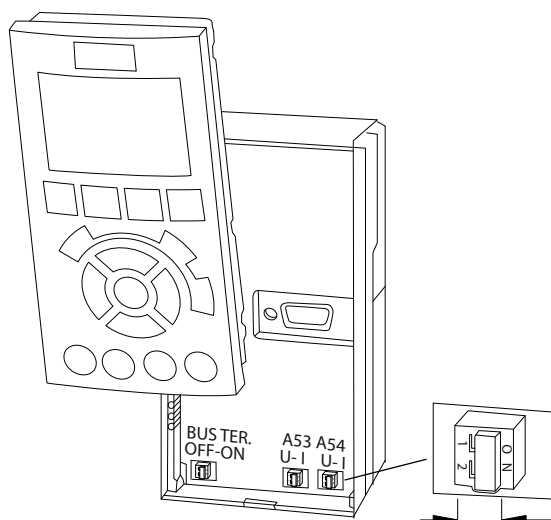
Illustration 5.22 Emplacement des commutateurs des bornes 53 et 54
