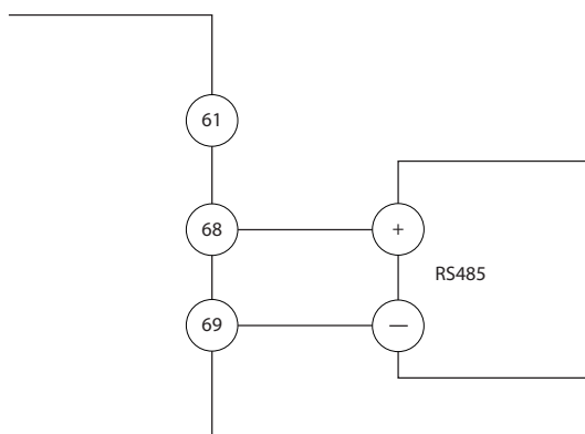
Illustration 5.21 Forbindelsesdiagram for seriel kommunikation
