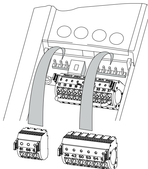
Illustration 5.17 Styreklemmeplaceringer
