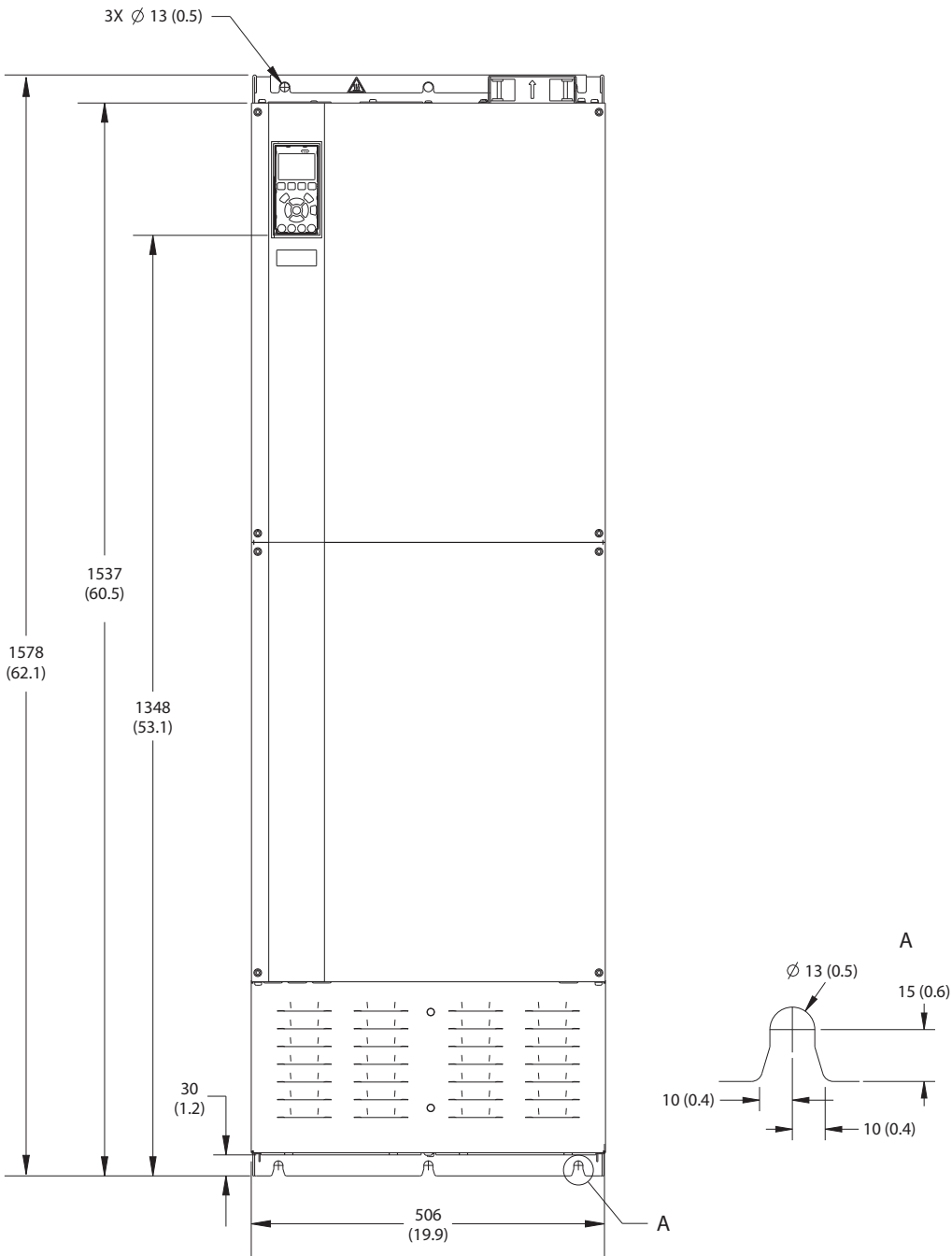
Abbildung 9.10 Frontansicht E3h
