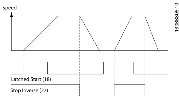
Abbildung 7.3 Puls-Start/Stop invers
