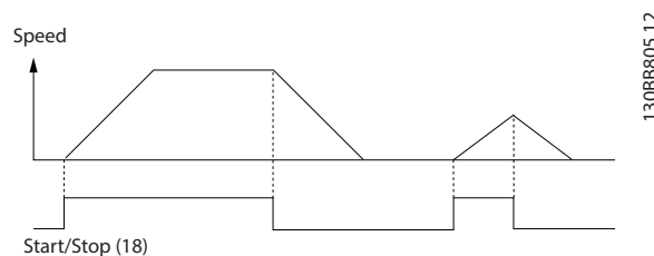
Ilustración 7.2 Orden de arranque/parada con Safe Torque Off
