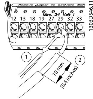
Çizim 5.20 Esnek Kontrol Tellerini Bağlama
