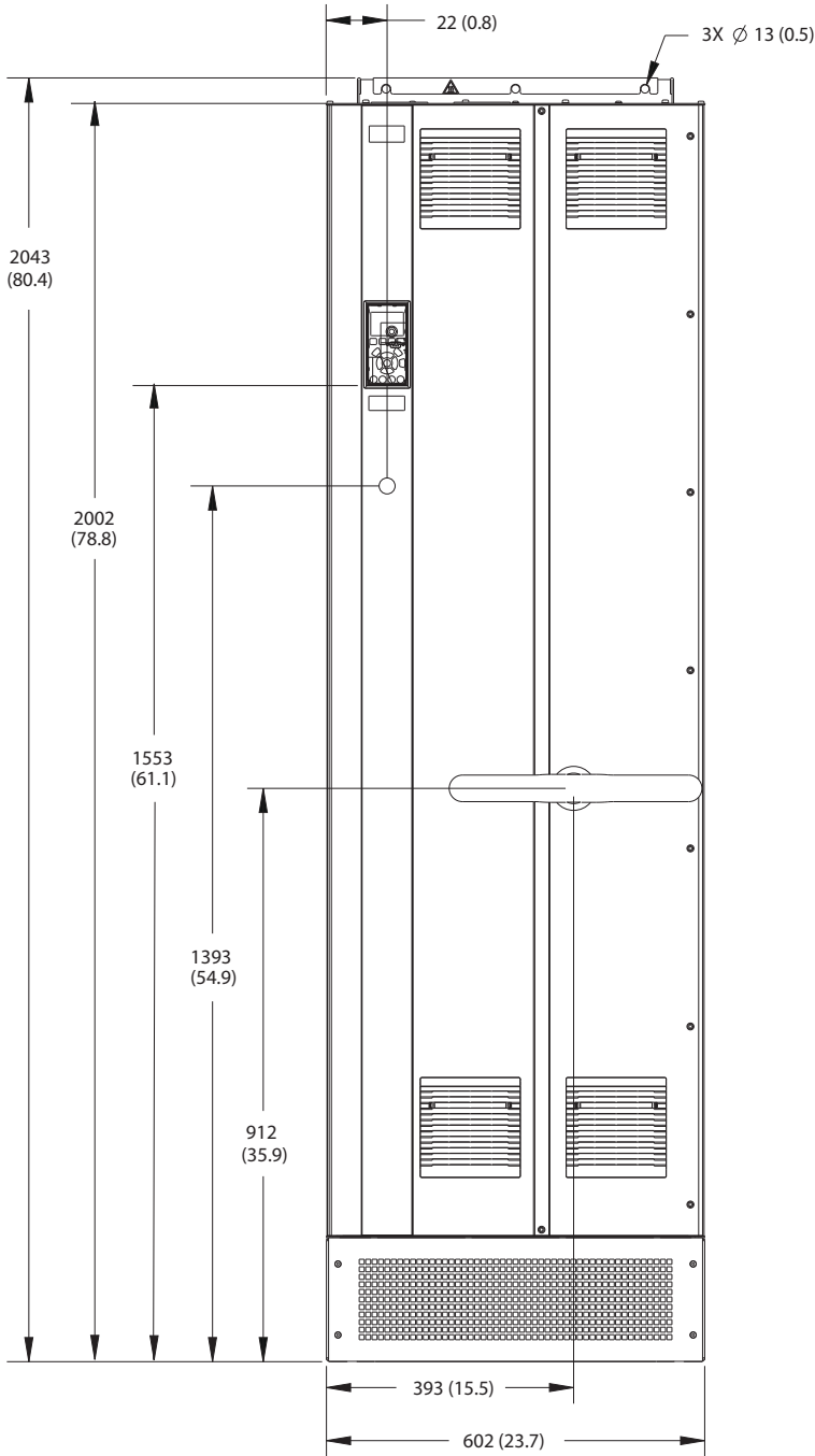
Çizim 9.2 E1h'nin Önden Görünümü
