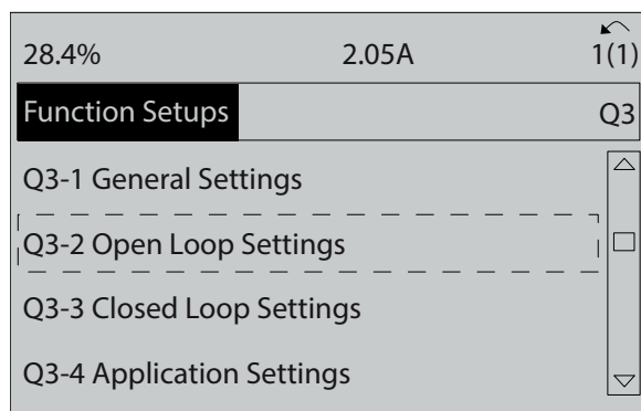
Ilustrația 6.4 Q3-2 Config bucl desch
