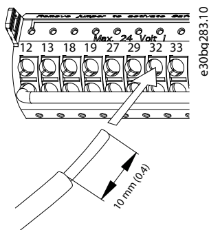
Ilustrația 5.19 Conectarea conductorilor de control solizi
