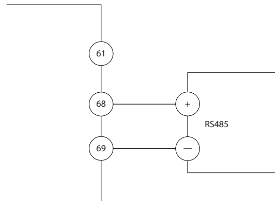
Ilustrația 5.21 Diagrama de cablare pentru comunicația serială
