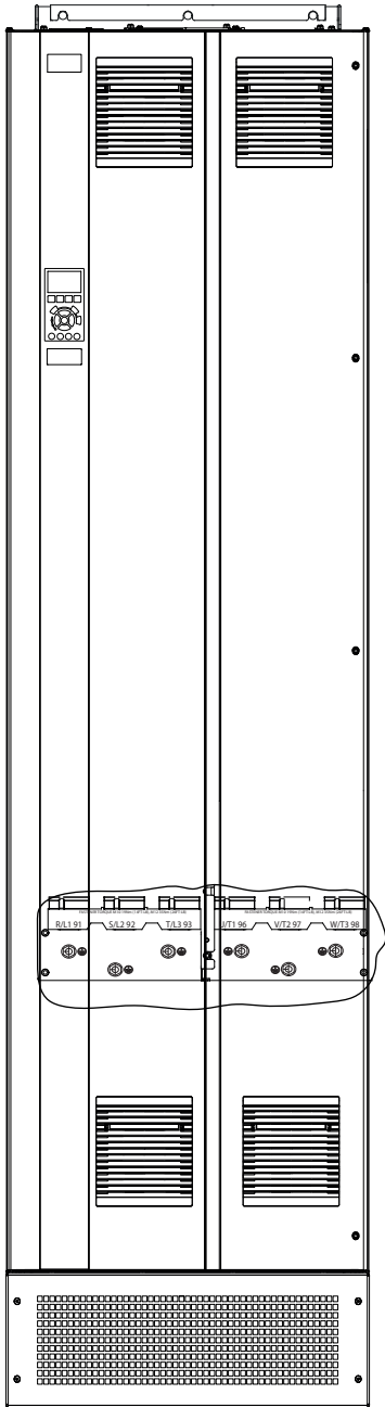
그림 5.5 접지 단자(예시 E1h). 자세한 단자 보기는 장을 5.7 단자 커수울(를) 참조하십시오.
