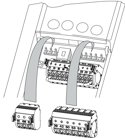
그림 5.17 제어 단자 위치
