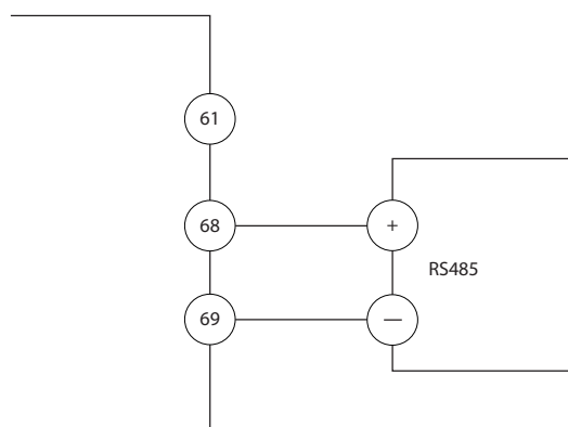
Ilustración 5.22 Diagrama de cableado de comunicación serie
