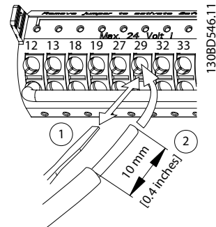
Ilustración 5.21 Conexión de los cables de control flexibles
