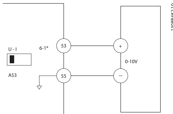
Ilustración 6.12 Ejemplo de cableado para el dispositivo externo que suministra una señal de control de 0-10 V
