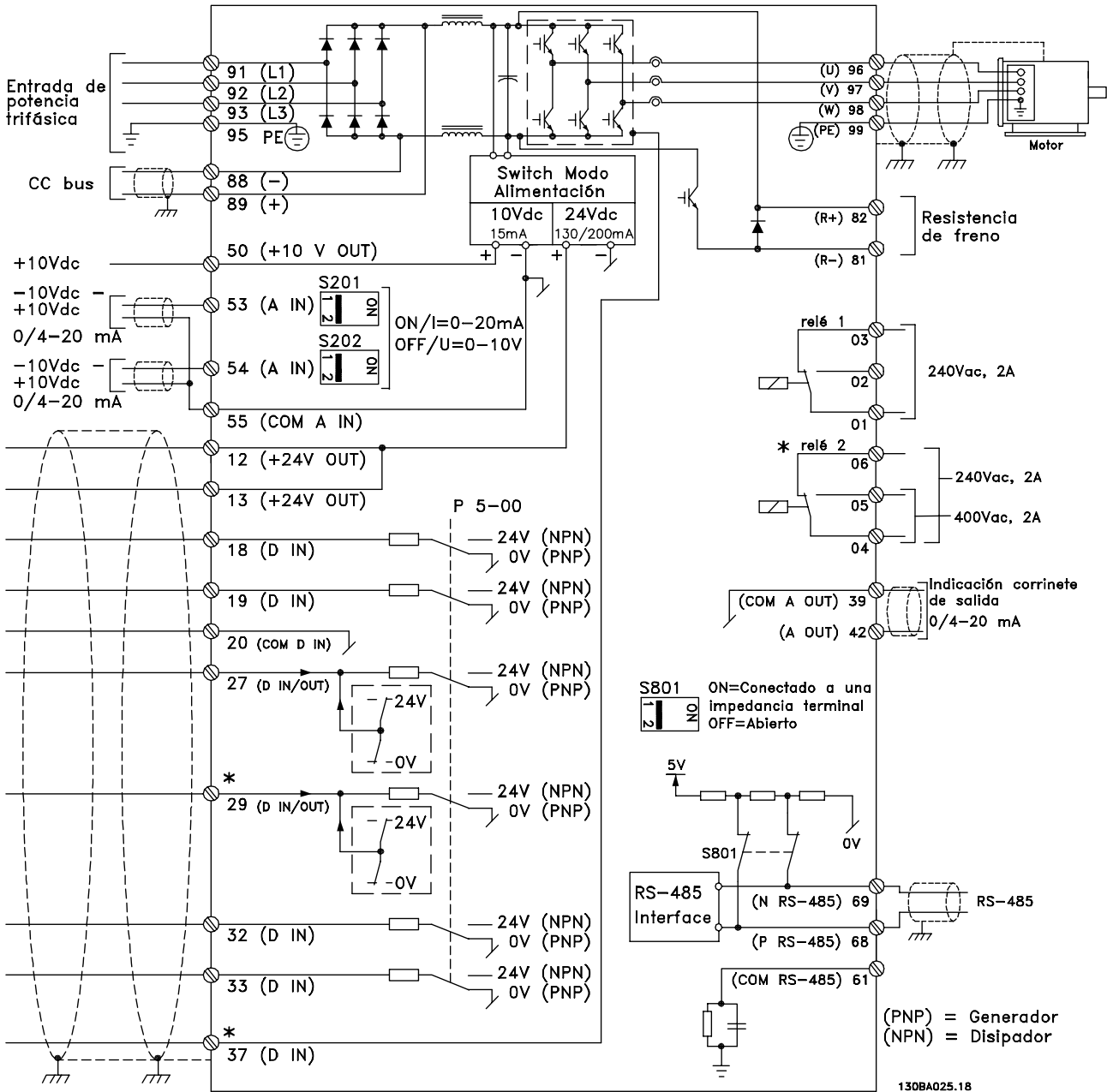
Ilustración 5.2 Esquema básico del cableado
