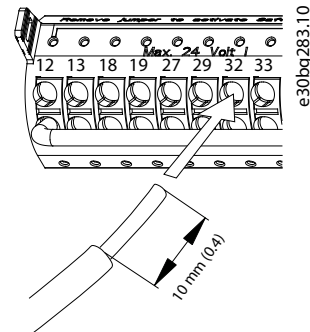
Ilustración 5.20 Conexión de los cables de control rígidos
