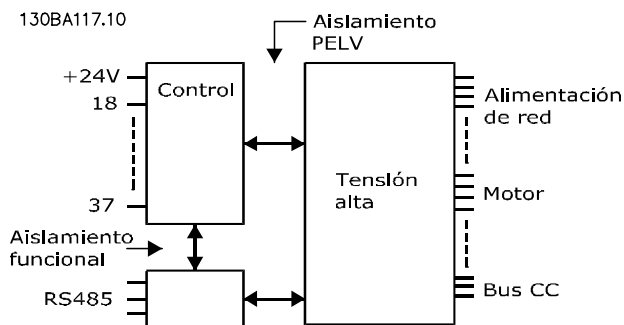
Ilustración 9.1 Aislamiento PELV
