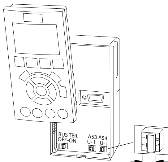
Ilustración 5.23 Ubicación de los conmutadores de los terminales 53 y 54
