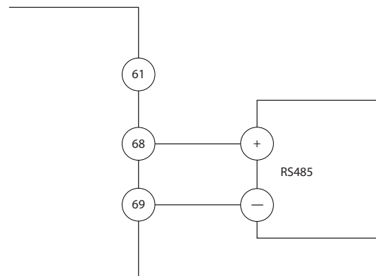
Afbeelding 5.22 Bedradingsschema voor seriële communicatie
