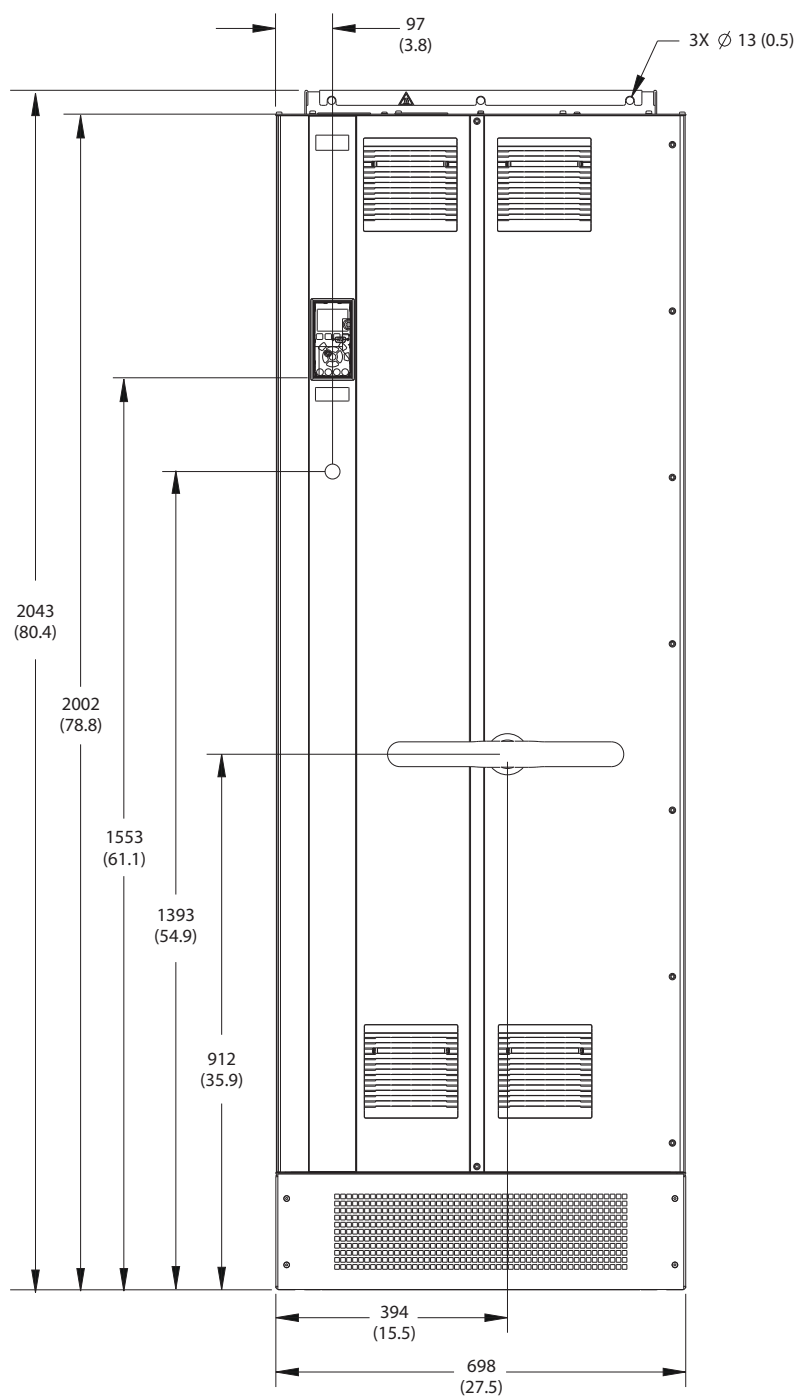
图 9.6 E2h 的正视图
