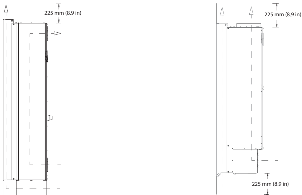
图 9.18 E1h/E2h (左) 和 E3h/E4h (右) 的标准气流配置
