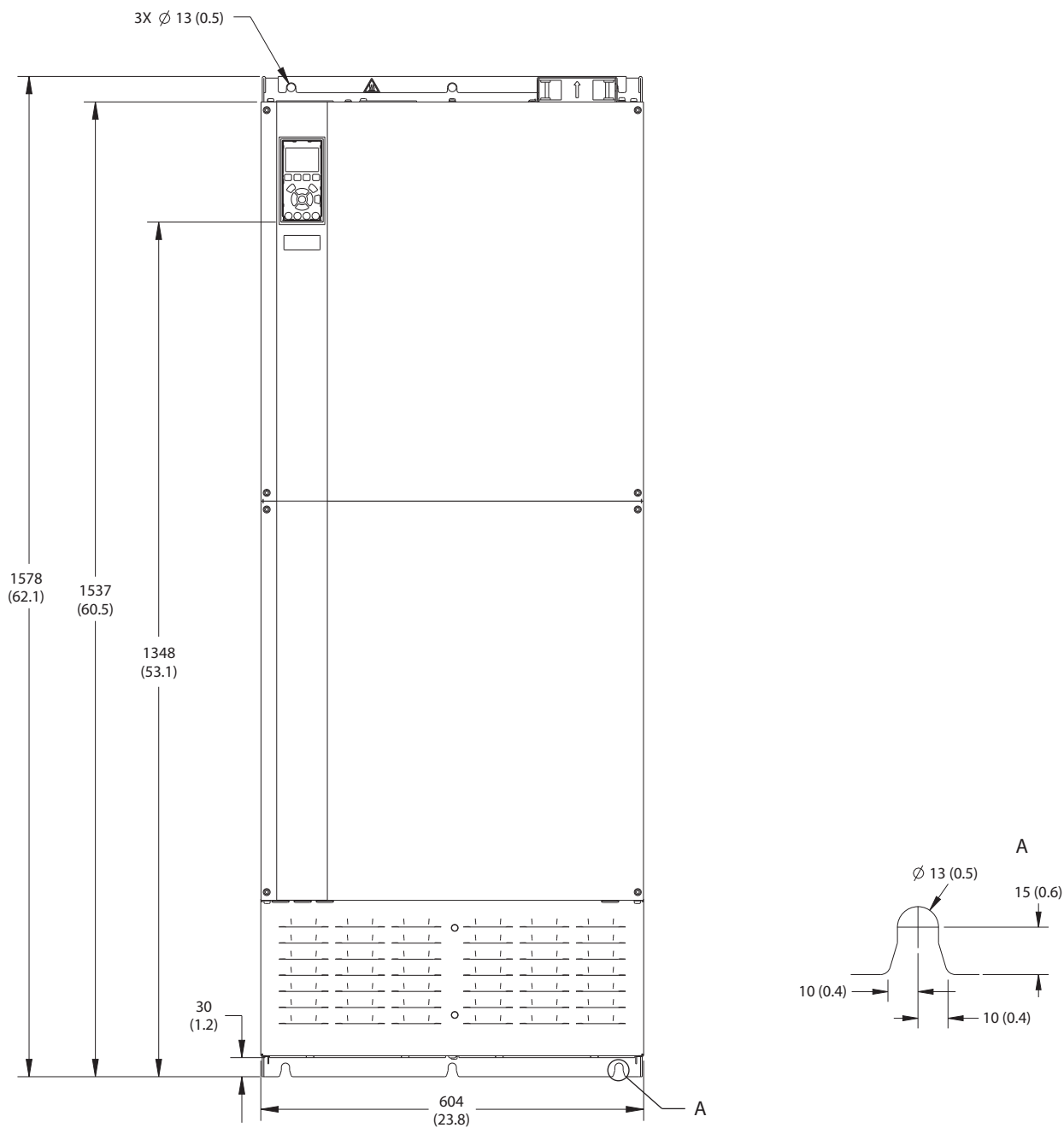
图 9.14 E4h 的正视图
