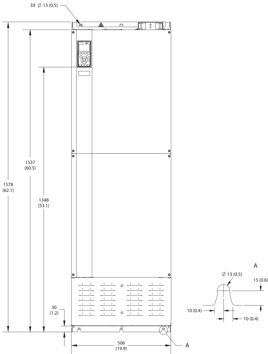
图 9.10 E3h 的正视图
