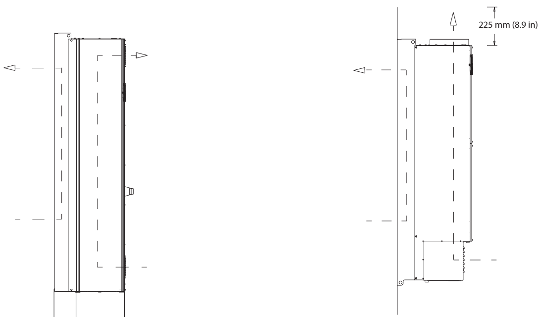
图 9.19 E1h/E2h (左) 和 E3h/E4h (右) 上通过后壁的可选气流配置
