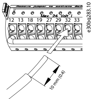
图 5.20 连接硬质控制线缆
