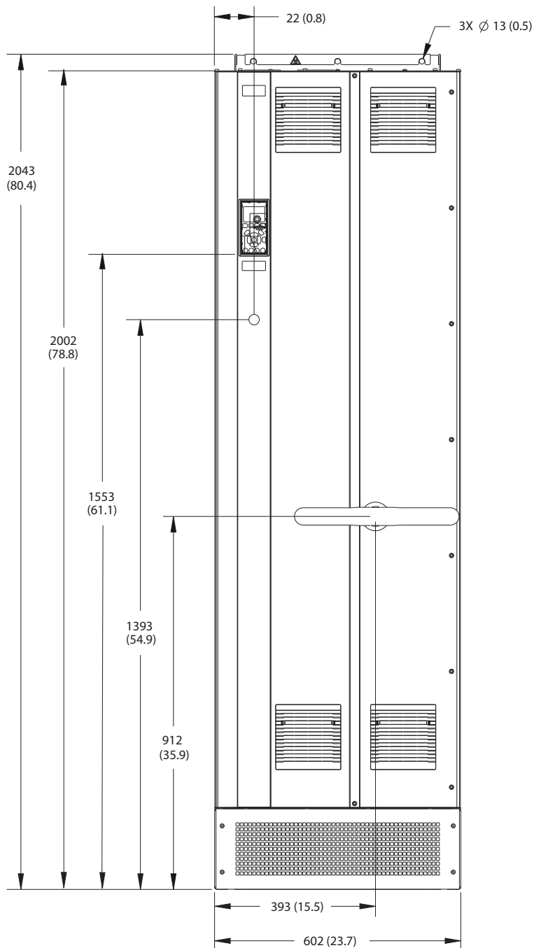
图 9.2 E1h 的正视图
