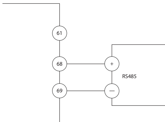
图 5.22 串行通讯接线图
