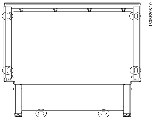
Ábra 4.3 A lábazzat és a padló közötti szerelési pontok
