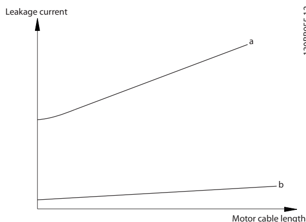
Рисунок 10.11 Влияние длины кабеля двигателя и типоразмера по мощности на ток утечки. Типоразмер по мощности a > типоразмера по мощности b
