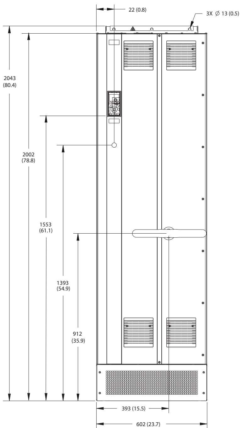
Рисунок 8.1 Вид спереди E1h
