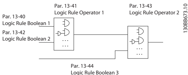
Рисунок 5.6 Логические соотношения
