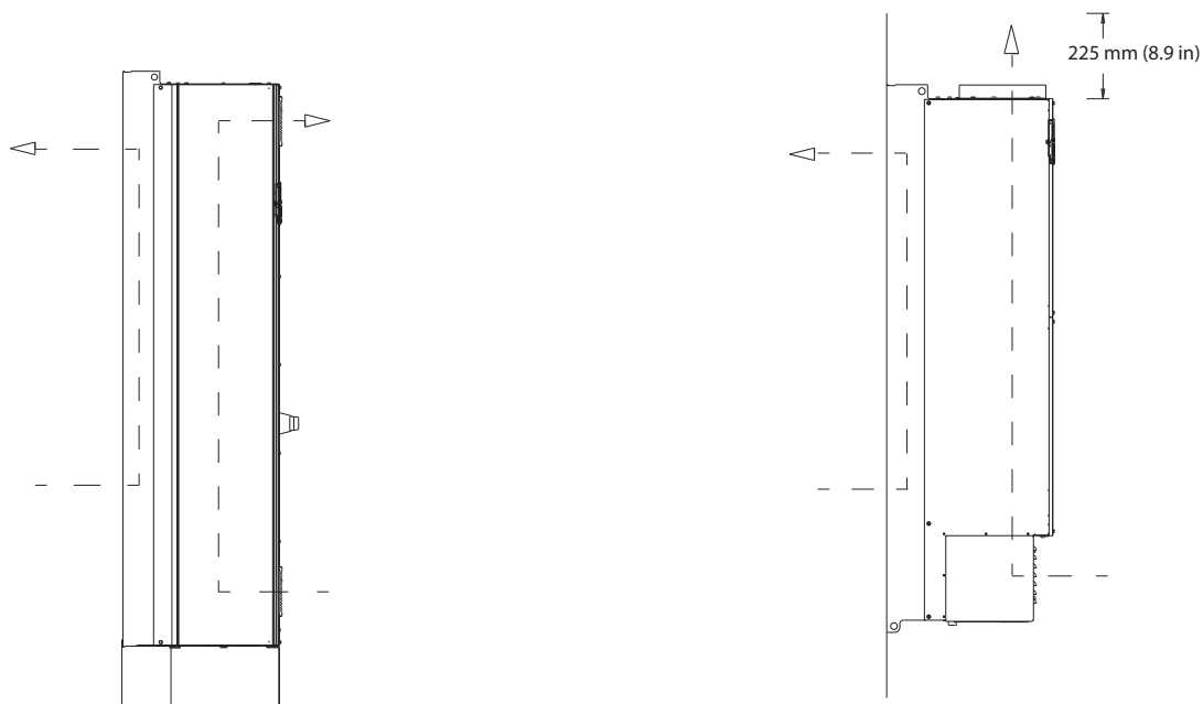
Рисунок 5.26 Вариант конфигурации воздушной циркуляции через заднюю стенку для E1h/E2h (слева) и E3h/E4h (справа)
