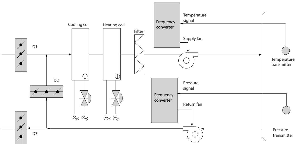
Рисунок 5.17 Использование преобразователя частоты в системе с постоянным объемом воздуха
