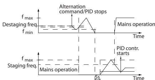
Рисунок 5.23 Чередование ведущего насоса
