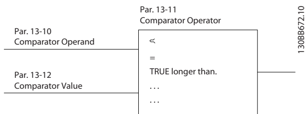
Рисунок 5.5 Компараторы
