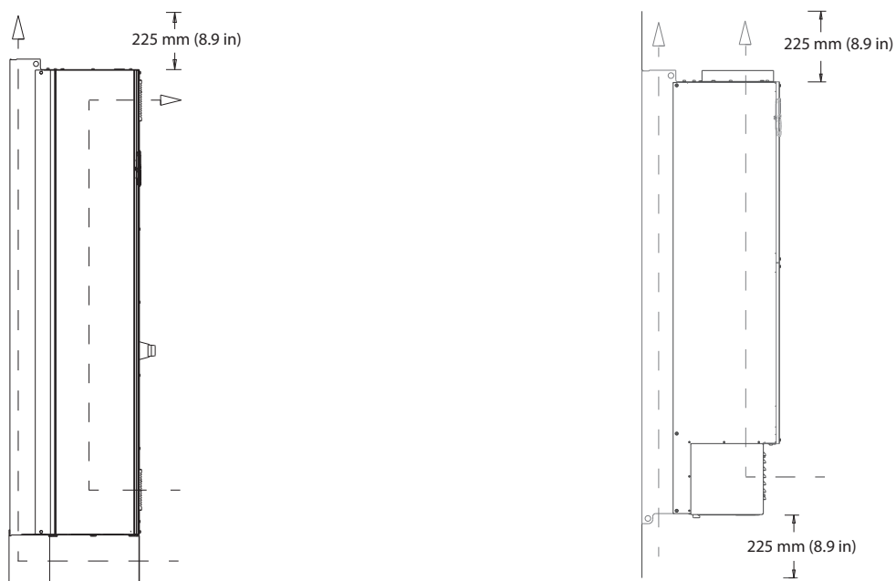
Рисунок 5.25 Стандартная конфигурация воздушной циркуляции для E1h/E2h (слева) и E3h/E4h (справа)
