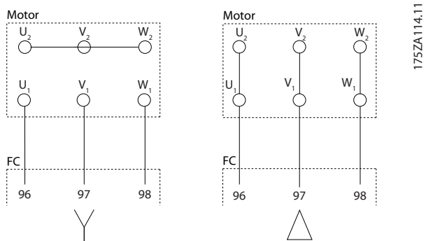
Ilustração 10.3 Conexão do cabo de motor
