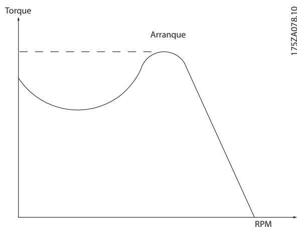
Ilustração 14.1 Gráfico de torque de segurança
