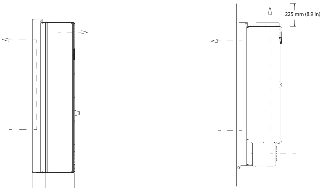
图 5.28 E1h/E2h (左) 和 E3h/E4h (右) 上通过后壁的可选气流配置
