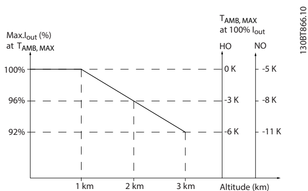
图 9.2 T_{AMB, MAX} 下基于海拔的输出电流降容
