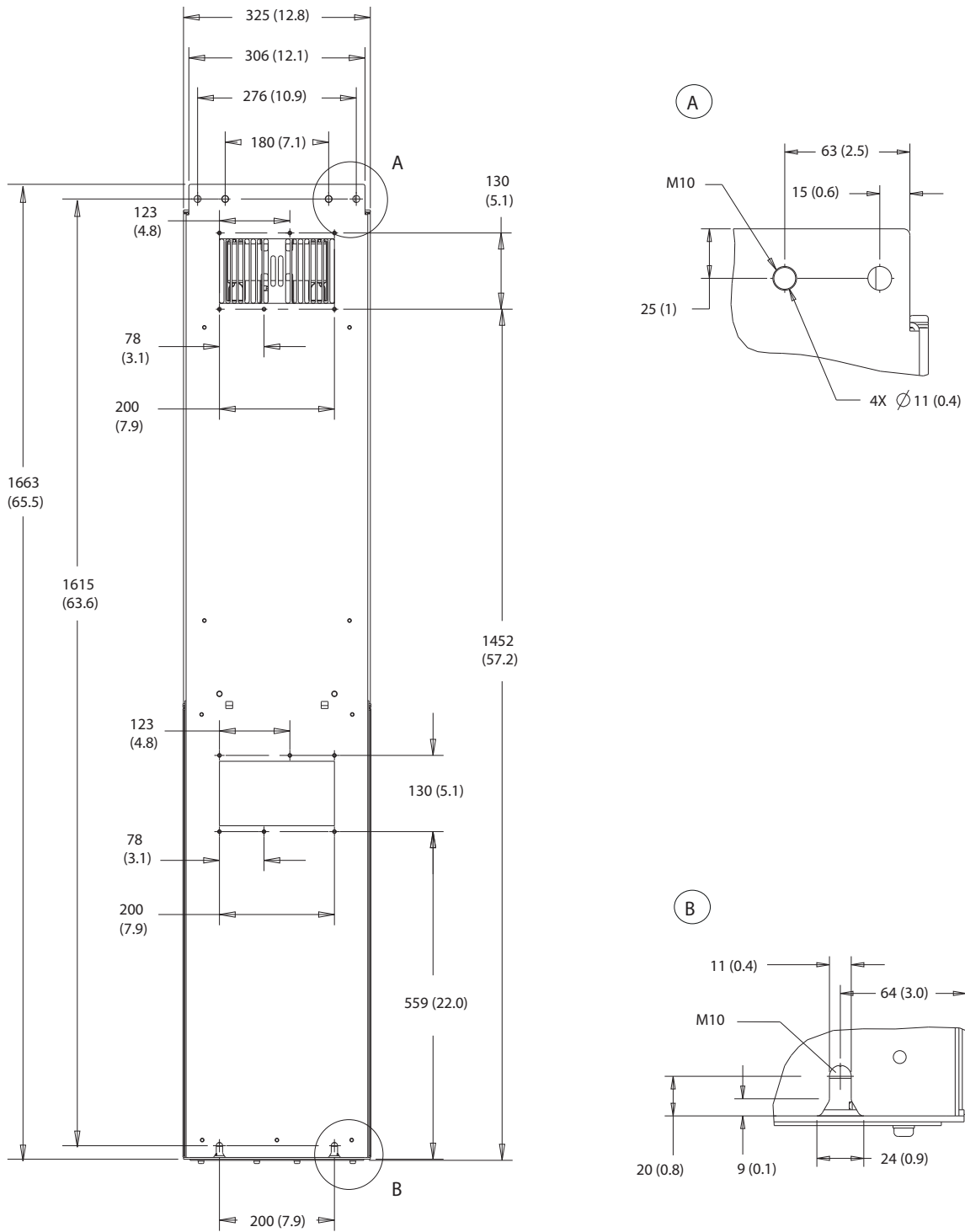
图 8.37 D6h 后视图
