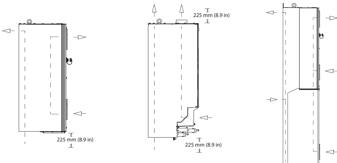
图 5.26 用于 D1h - D8h 机箱的背部风道冷却套件的可选气流配置。
