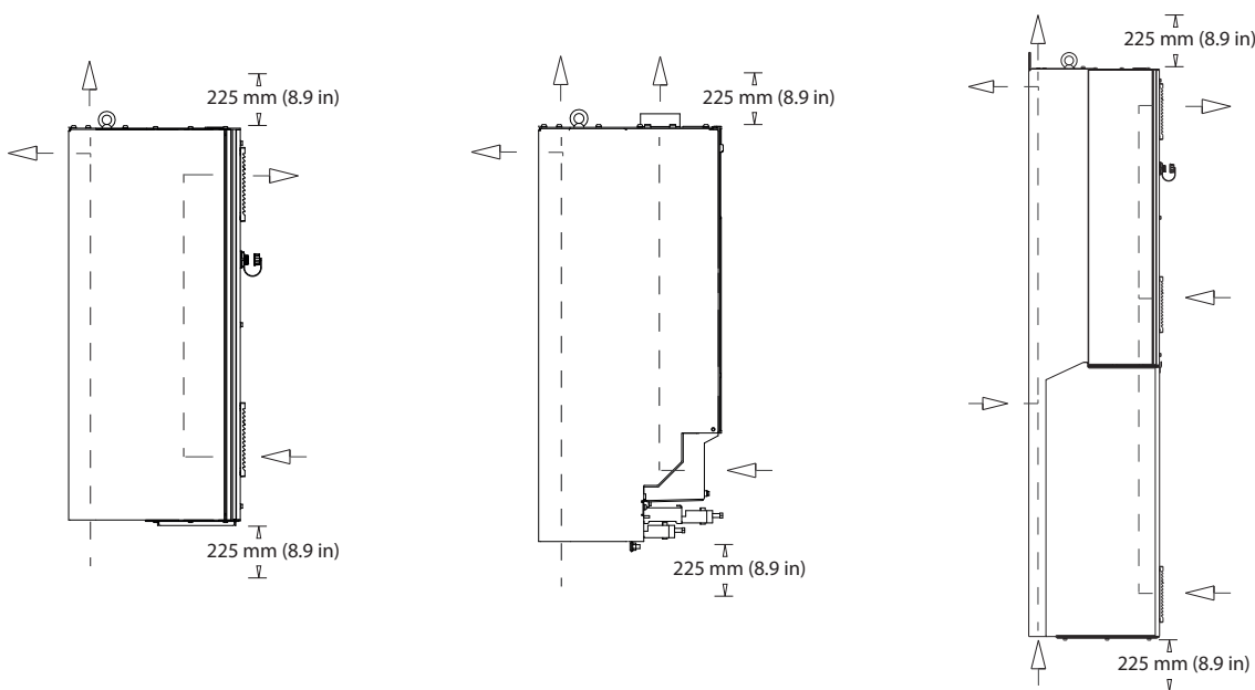
图 5.25 机箱 D1h/D2h (左)、D3h/D4h (中) 和 D5h - D8h (右) 的标准气流配置。
