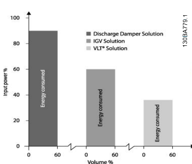
图 5.10 三种常见节能系统
