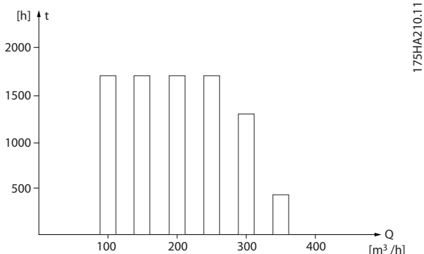
图 5.11 一年的流量分布
