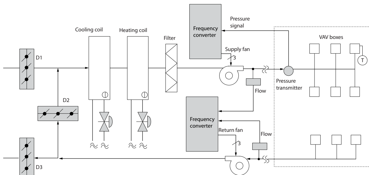
图 5.16 变风量系统中使用的变频器
