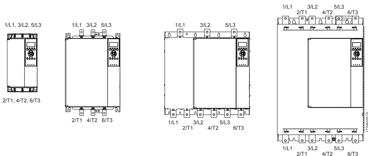
Ilustracja 4.3 Modele z wewnętrznym obejściem (od MCD5-0021B do MCD5-0105B, od MCD5-0131B do MCD5-0215B, od MCD5-0245B do MCD5-0396B, od MCD5-0469B do MCD5-0961B)
