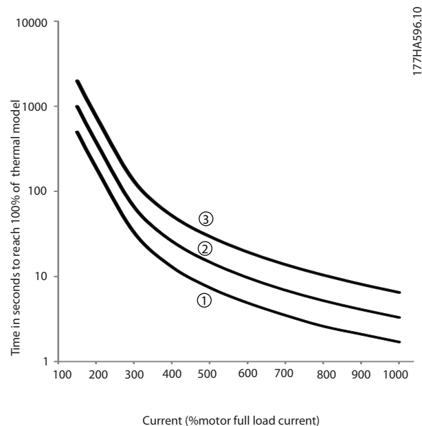
Ilustracja 5.1 Stopień ochrony w porównaniu z przeciążeniem
