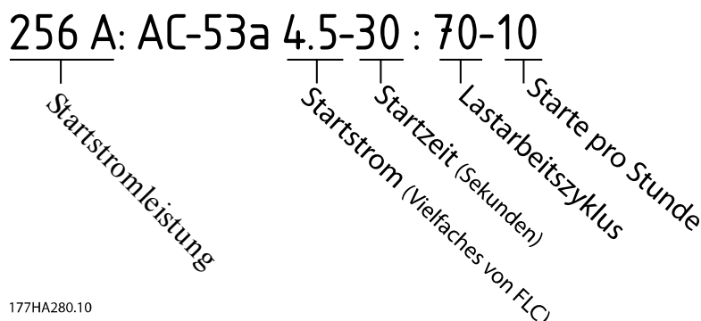
Abbildung 4.20 AC-53 Nennwerte für Dauerbetrieb
