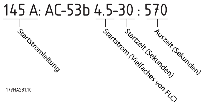
Abbildung 4.19 AC-53 Nennwerte für überbrückten Betrieb
