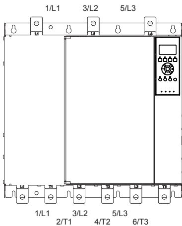
Abbildung 4.5 MCD5-0245B bis MCD5-0396B, 245–396 A
