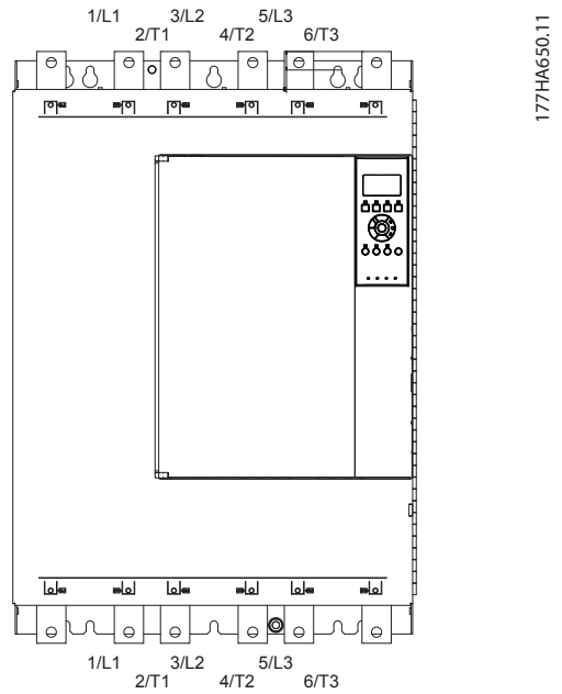
Abbildung 4.6 MCD5-0469B bis MCD5-0961B, 469–961 A
