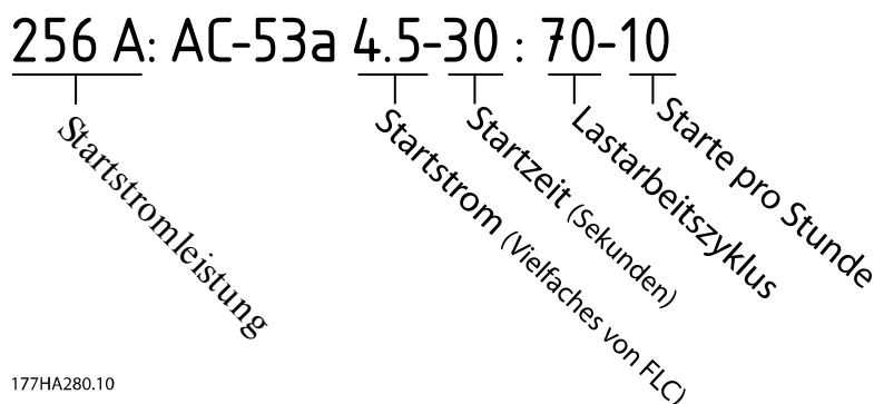
Abbildung 4.18 AC-53 Nennwerte für Dauerbetrieb
