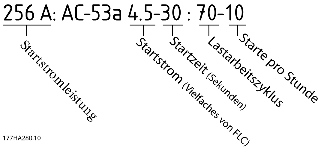
Abbildung 4.18 AC-53 Nennwerte für Dauerbetrieb
