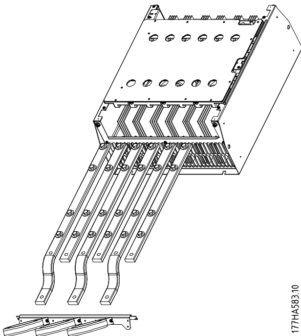
Abbildung 12.2 Sammelschienen
