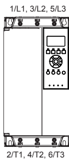
Abbildung 4.3 MCD5-0021B bis MCD5-0105B, 21–105 A
