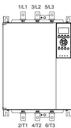
Abbildung 4.4 MCD5-0131B bis MCD5-0215B, 131–215 A
