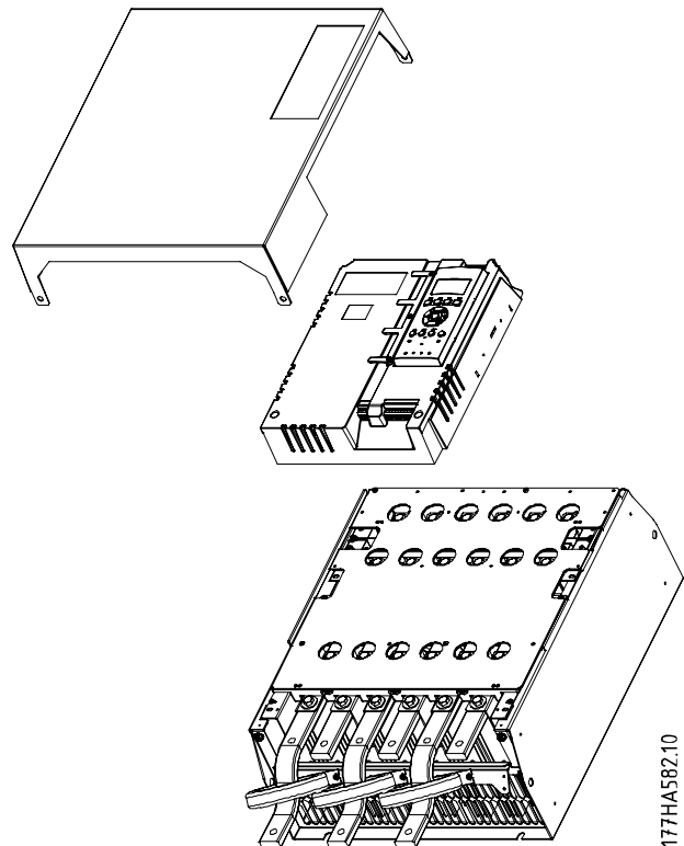
Abbildung 12.1 Entfernen der Frontabdeckung und des LCP
