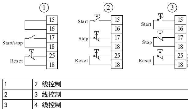
图 4.2 2、3 和 4 线控制
