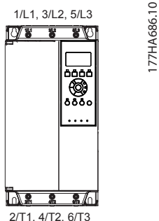
图 4.3 MCD5-0021B 至 MCD5-0105B, 21 - 105 A
