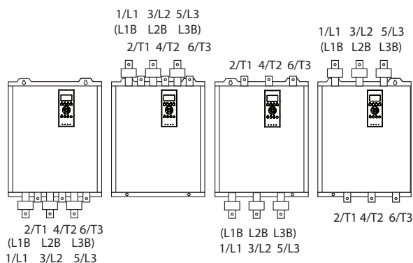
图 4.8 旁路端子的位置, MCD5-0360C 至 MCD5-1600C, 360 - 1600 A
