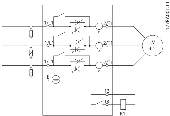
图 11.1 带有电涌保护套件的系统
